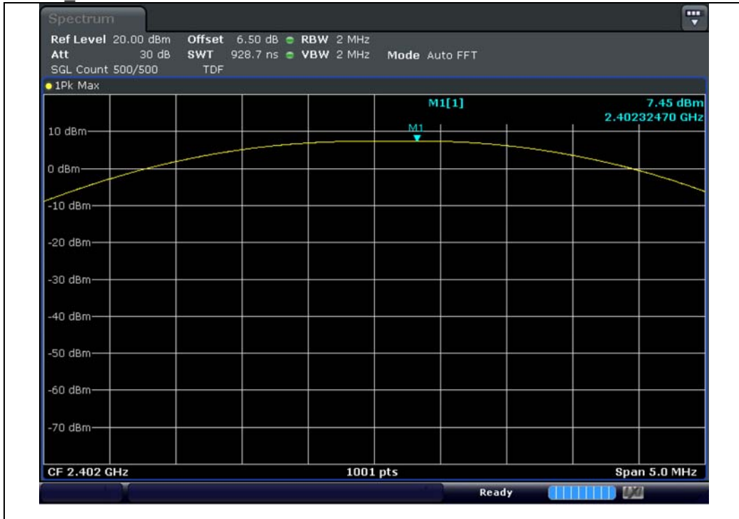
GFSK 2 402 MHz
