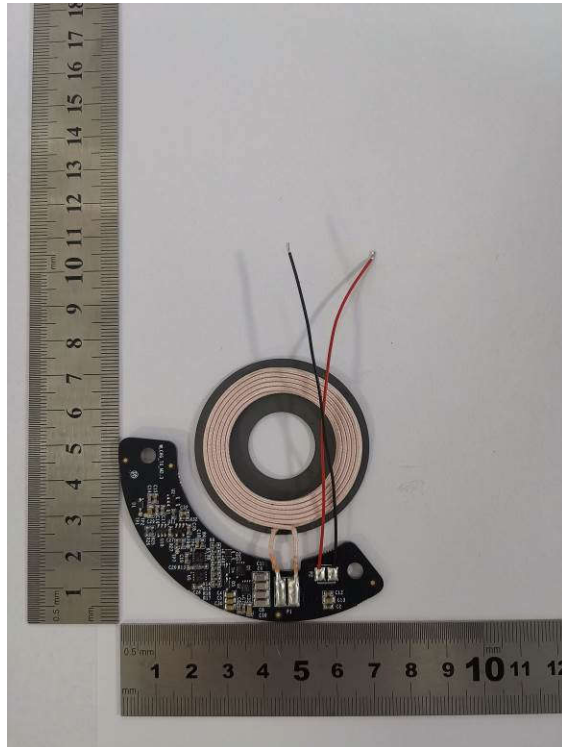
(31) EUT Photo (WLCHG_TX_V2.3)
