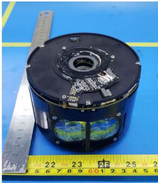
(24) EUT Photo (Pandar40 2.0)
