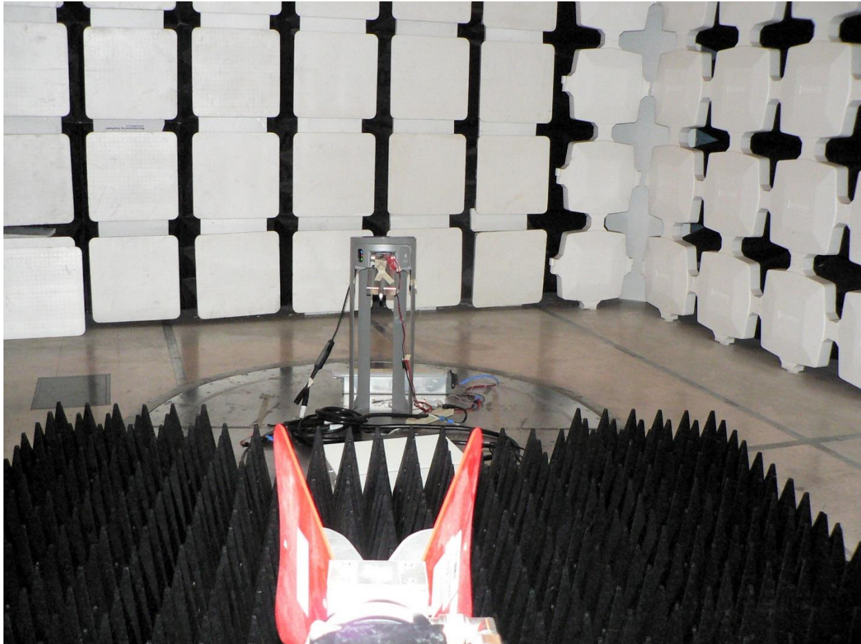
LYFT17 1-18GHz Emissions
