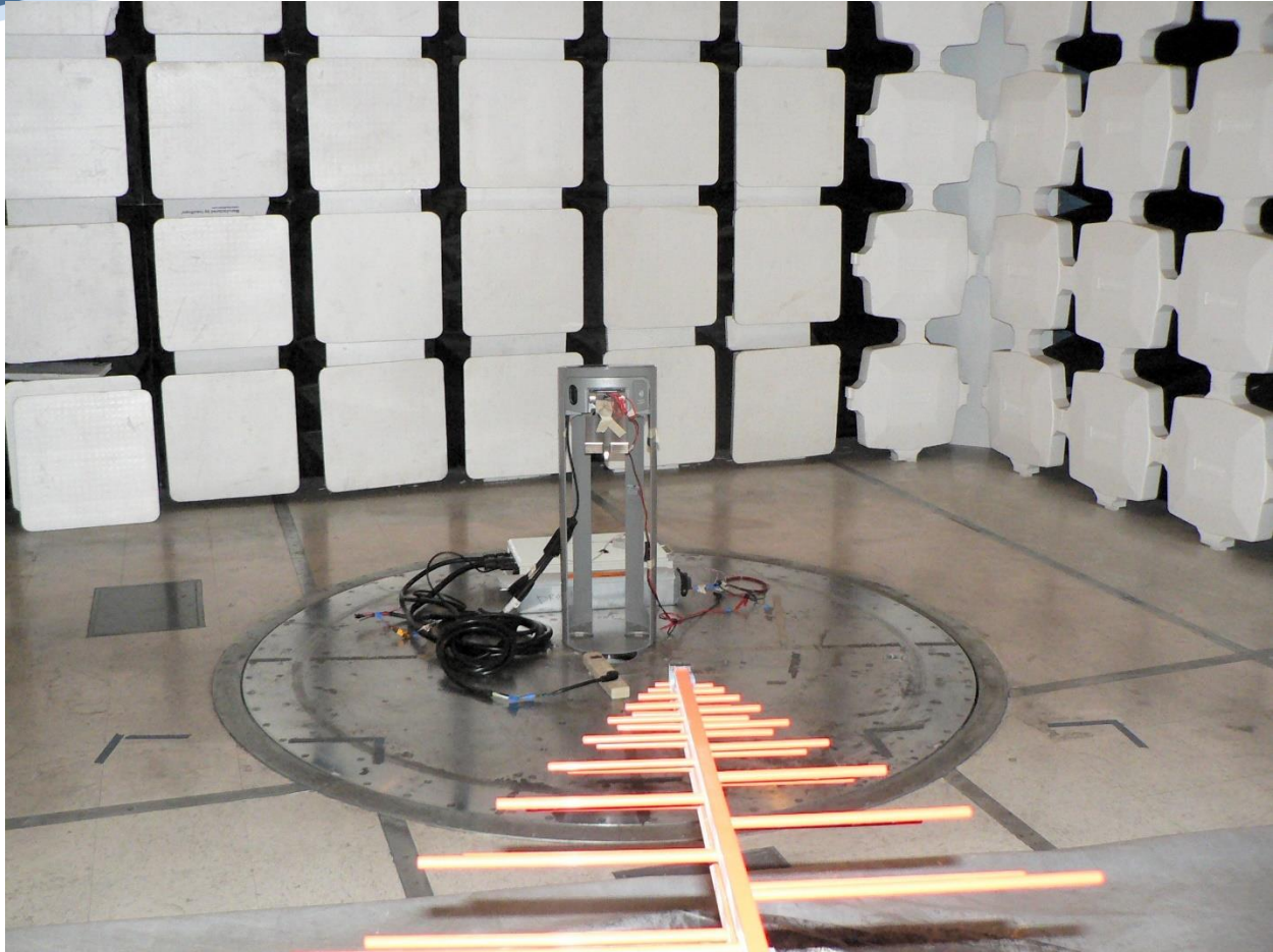
LYFT17 30-1000MHz Emissions
