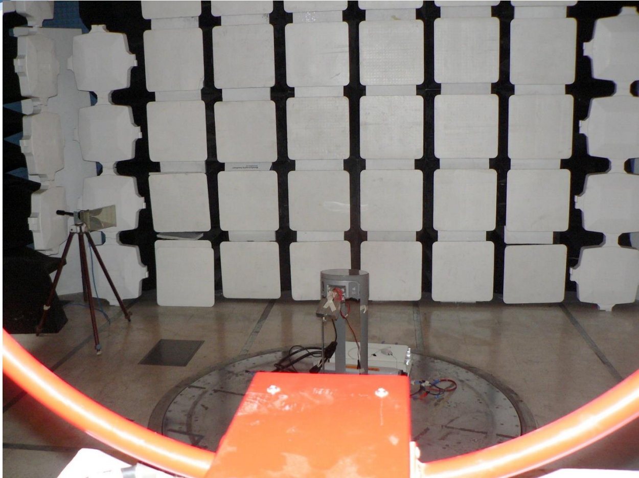
LYFT17 9k-30MHz Emissions
