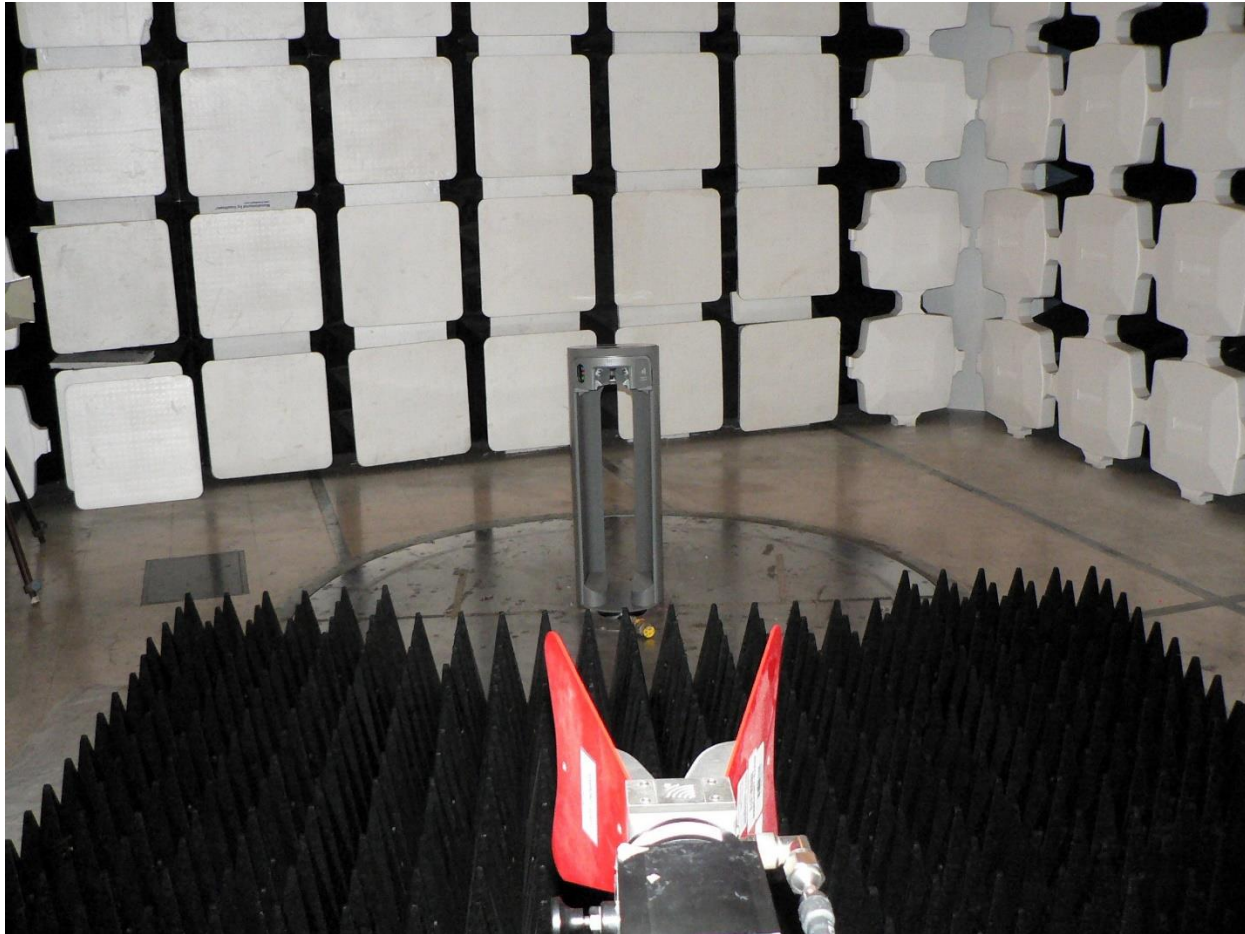
LYFT17 Solar DVT 1-18GHz Emissions
