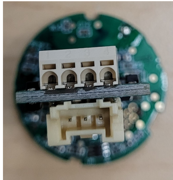
Bottom Side
