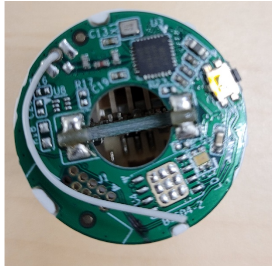
Bottom Side
