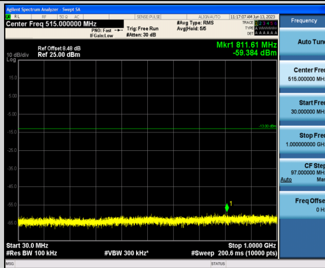
Band66-5MHz-16QAM-132647-1-0-Low-30-1000--59.38-PASS
