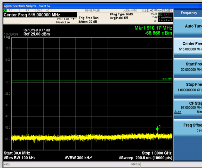
Band66-3MHz-16QAM-131987-1-0-Low-30-1000--58.87-PASS
