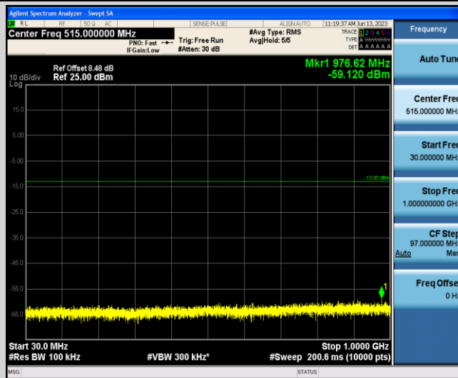
Band66-10MHz-QPSK-132622-1-0-Low-30-1000--59.12-PASS
