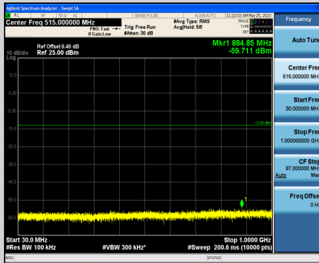
Band66-3MHz-QPSK-132322-1-0-Low-30-1000--59.71-PASS
