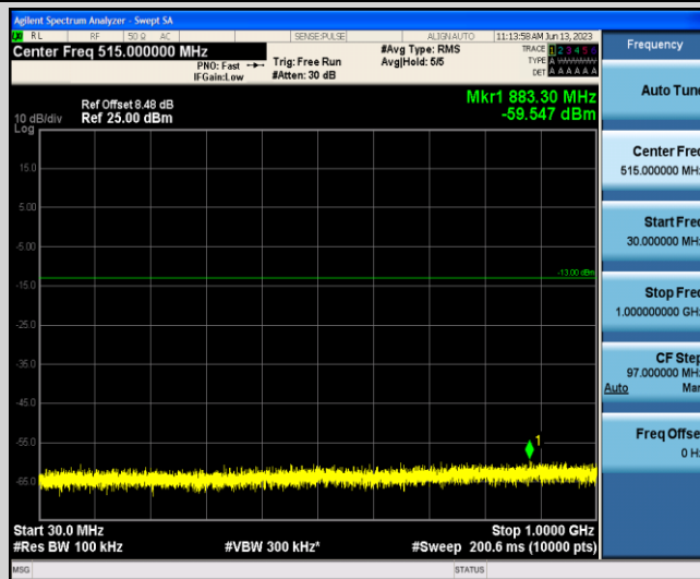
Band66-3MHz-QPSK-132657-1-0-Low-30-1000--59.55-PASS
