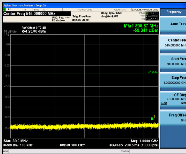
Band66-10MHz-QPSK-132022-1-0-Low-30-1000--59.04-PASS
