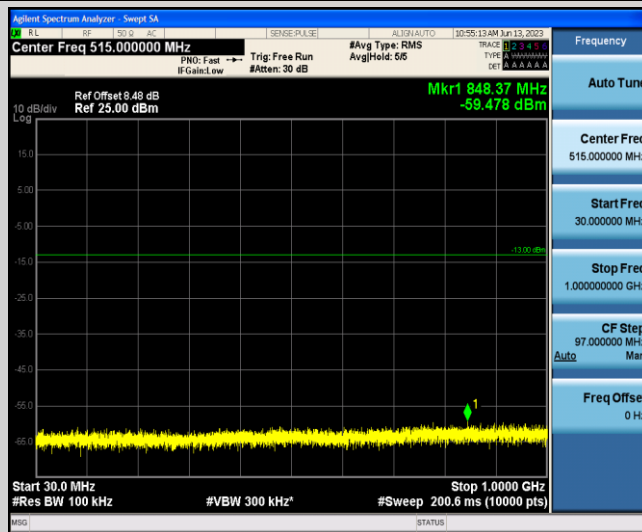
Band4-3MHz-QPSK-20175-1-0-Low-30-1000--59.48-PASS
