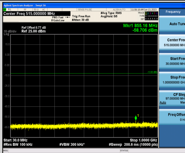
Band4-20MHz-16QAM-20050-1-0-Low-30-1000--58.71-PASS
