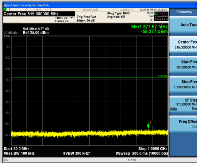
Band4-20MHz-QPSK-20050-1-0-Low-30-1000--59.38-PASS
