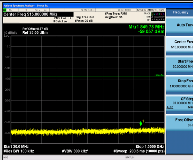
Band4-10MHz-QPSK-20000-1-0-Low-30-1000--59.06-PASS
