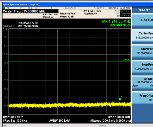
Band4-5MHz-QPSK-19975-1-0-Low-30-1000--59.46-PASS
