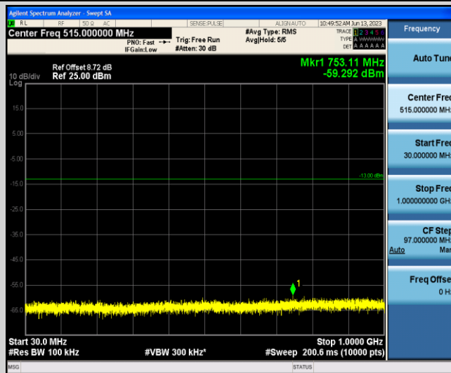
Band2-20MHz-QPSK-18700-1-0-Low-30-1000--59.29-PASS
