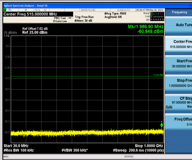
Band2-10MHz-QPSK-18900-1-0-Low-30-1000--60.85-PASS
