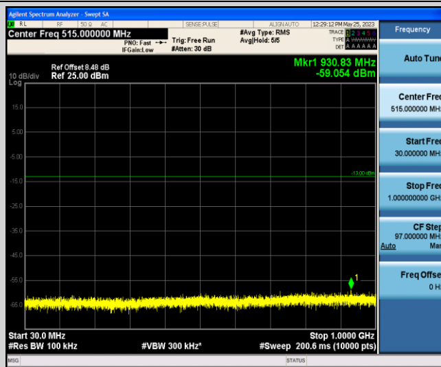
Band4-1.4MHz-QPSK-20175-1-0-Low-30-1000--59.05-PASS
