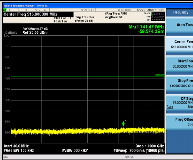
Band4-1.4MHz-16QAM-19957-1-0-Low-30-1000--59.57-PASS
