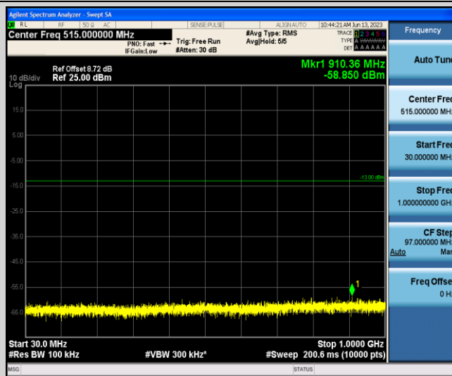
Band2-1.4MHz-QPSK-18900-1-0-Low-30-1000--58.85-PASS
