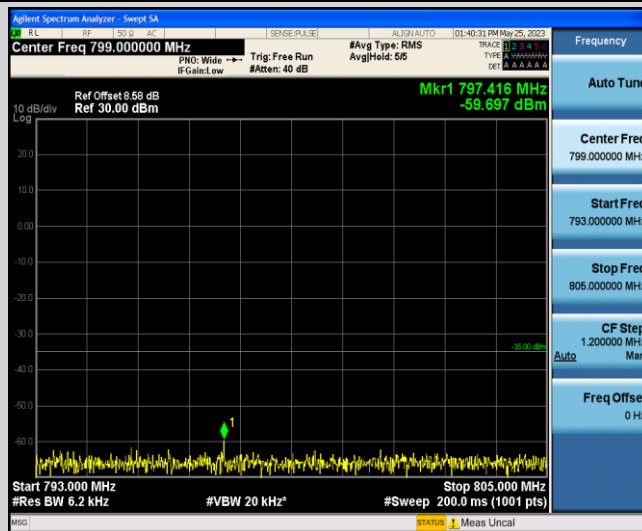
Band13-10MHz-QPSK-23230-1-0-Low-793-805--59.7-PASS
