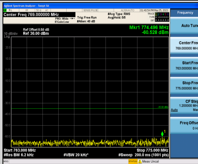
Band13-10MHz-16QAM-23230-1-0-Low-763-775--60.53-PASS
