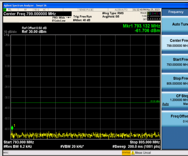
Band13-5MHz-QPSK-23255-1-0-Low-793-805--61.71-PASS
