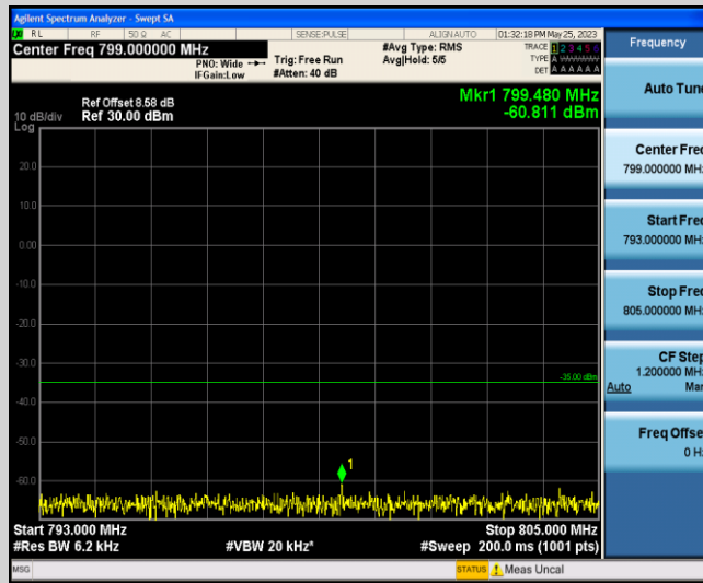
Band13-5MHz-16QAM-23230-1-0-Low-793-805--60.81-PASS
