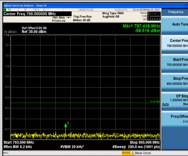
Band13-10MHz-16QAM-23230-1-0-Low-793-805--59.52-PASS
