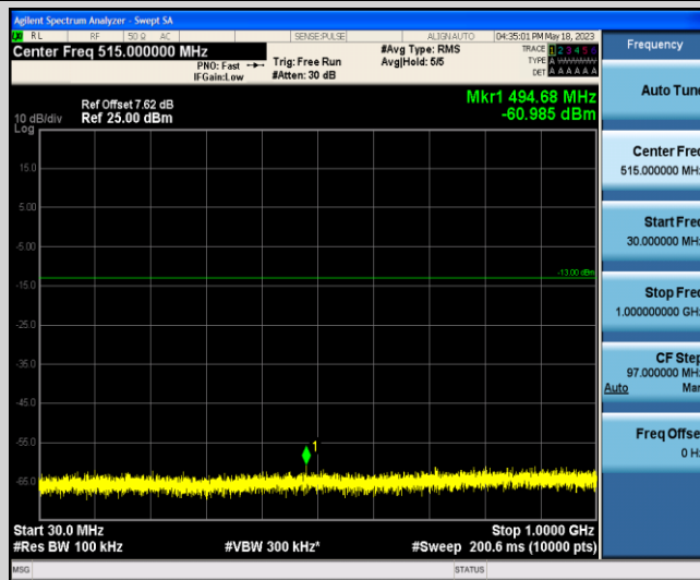
Band2-3MHz-16QAM-18900-1-0-Low-30-1000--60.99-PASS
