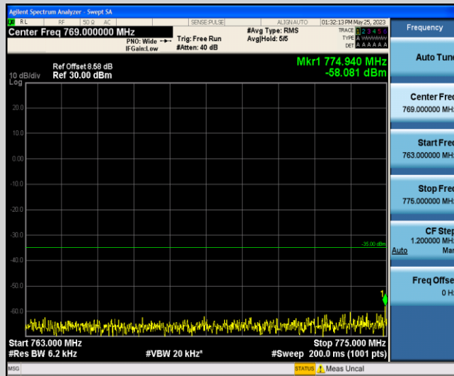
Band13-5MHz-16QAM-23230-1-0-Low-763-775--58.08-PASS
