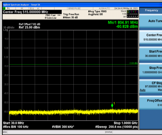
Band2-3MHz-QPSK-18900-1-0-Low-30-1000--60.83-PASS
