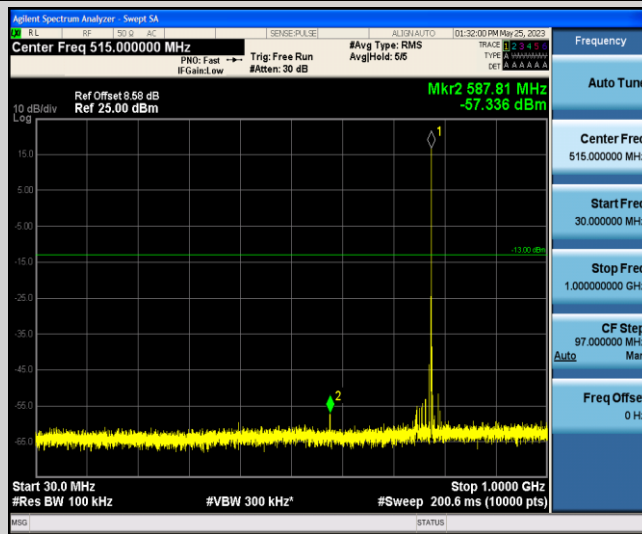
Band13-5MHz-16QAM-23230-1-0-Low-30-1000--57.34-PASS
