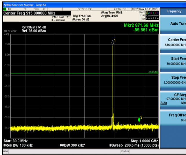
Band12-10MHz-QPSK-23060-1-0-Low-30-1000--59.86-PASS
