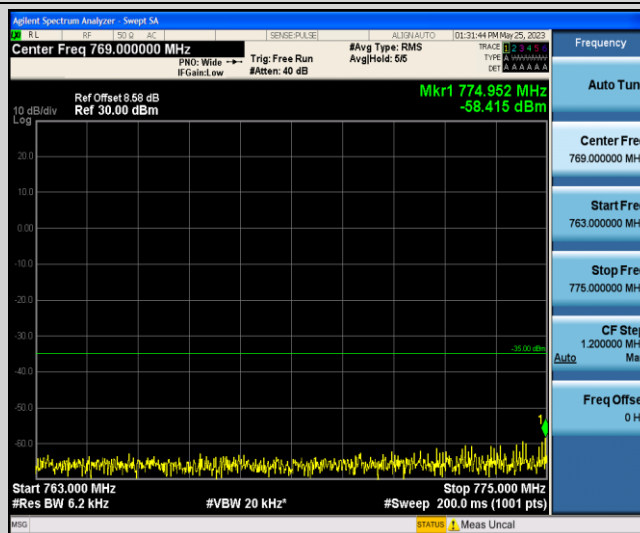
Band13-5MHz-QPSK-23230-1-0-Low-763-775--58.42-PASS
