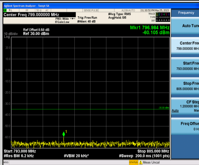
Band13-5MHz-QPSK-23205-1-0-Low-793-805--60.11-PASS
