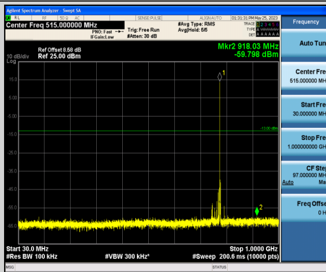
Band13-5MHz-QPSK-23230-1-0-Low-30-1000--59.8-PASS
