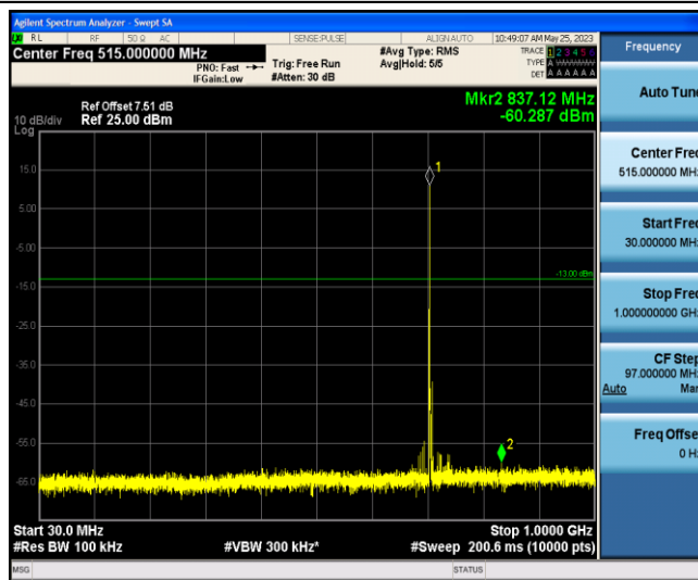
Band12-5MHz-QPSK-23155-1-0-Low-30-1000--60.29-PASS
