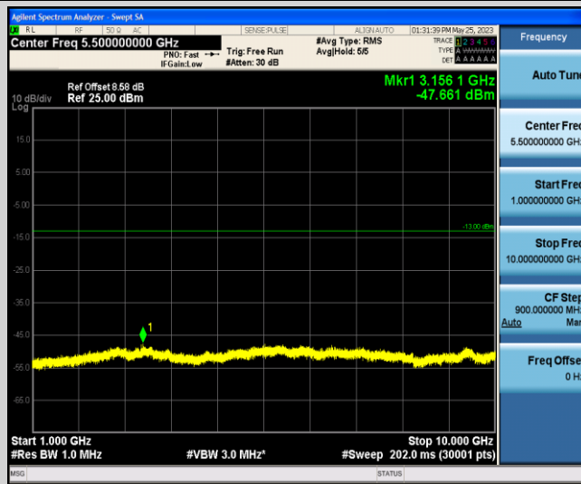
Band13-5MHz-QPSK-23230-1-0-Low-1000-10000--47.66-PASS
