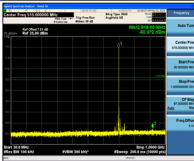
Band12-10MHz-QPSK-23130-1-0-Low-30-1000--60.37-PASS
