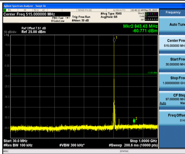
Band12-3MHz-QPSK-23165-1-0-Low-30-1000--60.77-PASS
