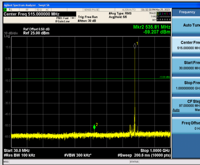
Band13-5MHz-QPSK-23255-1-0-Low-30-1000--59.21-PASS
