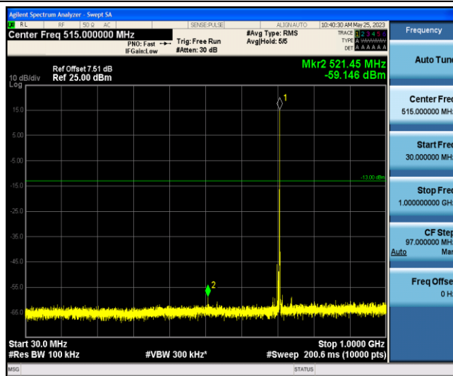
Band12-3MHz-16QAM-23165-1-0-Low-30-1000--59.15-PASS
