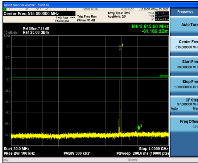
Band12-1.4MHz-QPSK-23017-1-0-Low-30-1000--61.19-PASS
