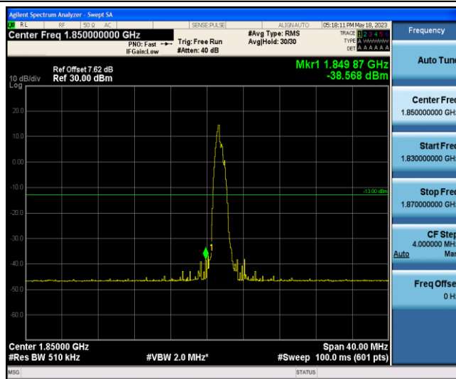
Band2-20MHz-QPSK-18700-1-0-Low--38.57-PASS
