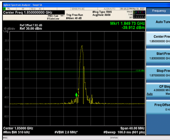
Band2-20MHz-16QAM-18700-1-0-Low--39.91-PASS
