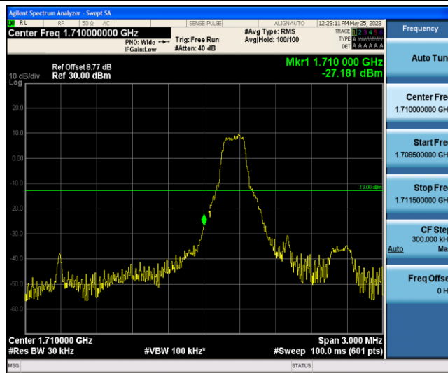
Band4-1.4MHz-QPSK-19957-1-0-Low--27.18-PASS
