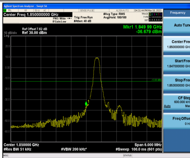
Band2-3MHz-QPSK-18615-1-0-Low--36.68-PASS
