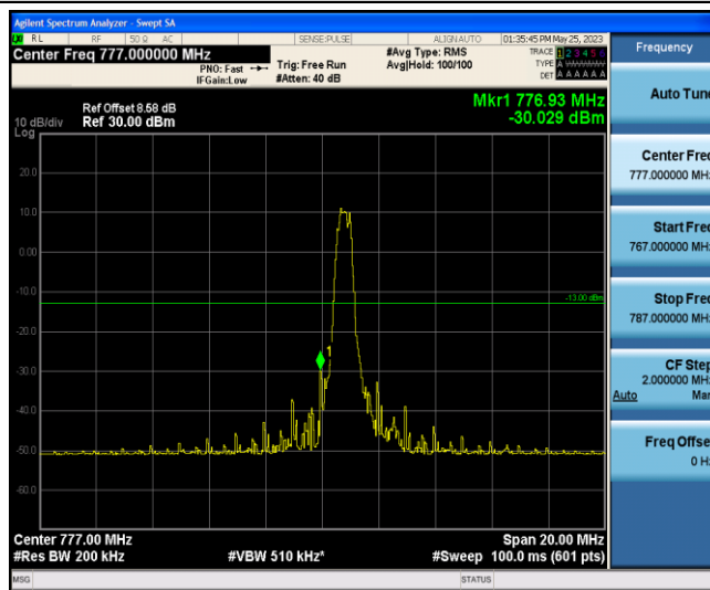
Band13-10MHz-QPSK-23230-1-0-Low--30.03-PASS
