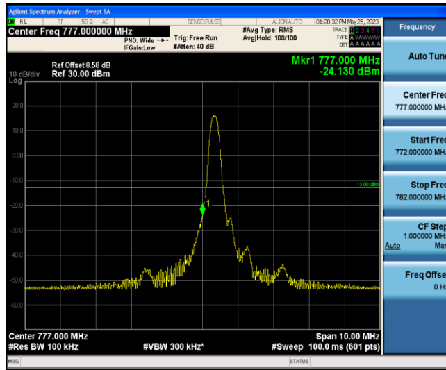
Band13-5MHz-16QAM-23205-1-0-Low--24.13-PASS
