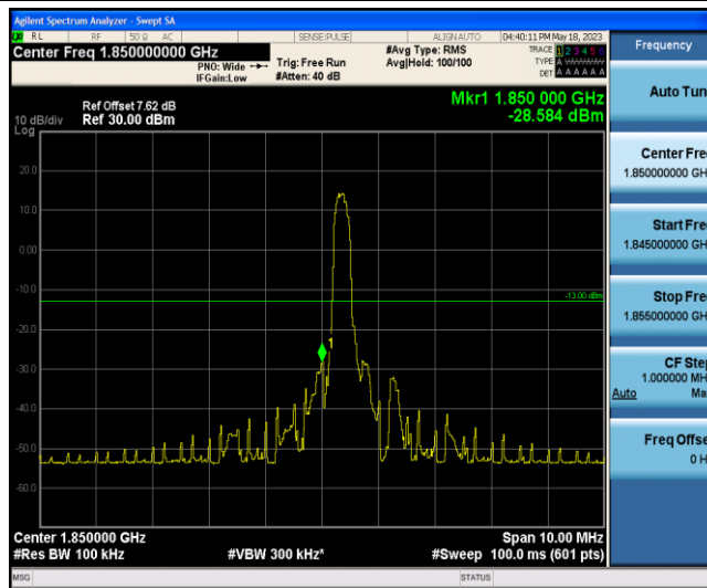
Band2-5MHz-QPSK-18625-1-0-Low--28.58-PASS
