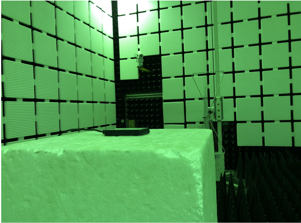
Fig. 1 (Below 1GHz)
