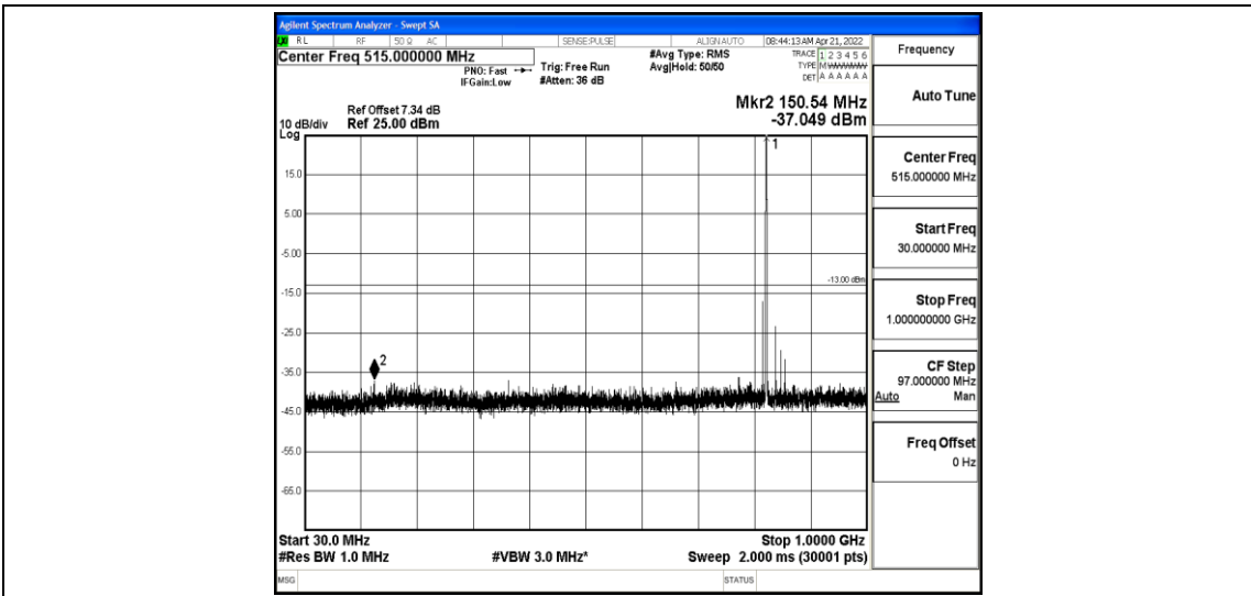
Band26-15MHz-QPSK-26865-1-0-Low-30-1000--37.05-PASS
