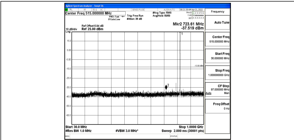
Band26-10MHz-16QAM-26840-1-0-Low-30-1000--37.52-PASS
