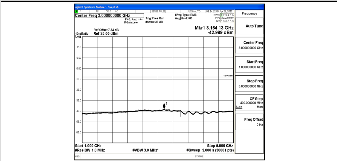
Band26-10MHz-QPSK-26915-1-0-Low-1000-5000--42.99-PASS
