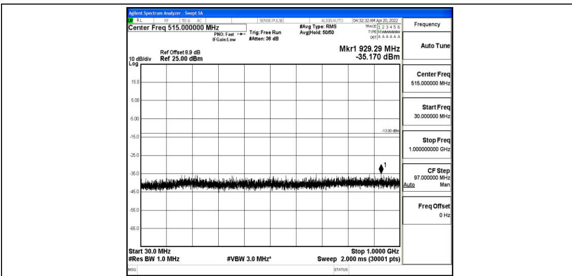
Band25-1.4MHz-QPSK-26047-1-0-Low-30-1000--35.17-PASS
