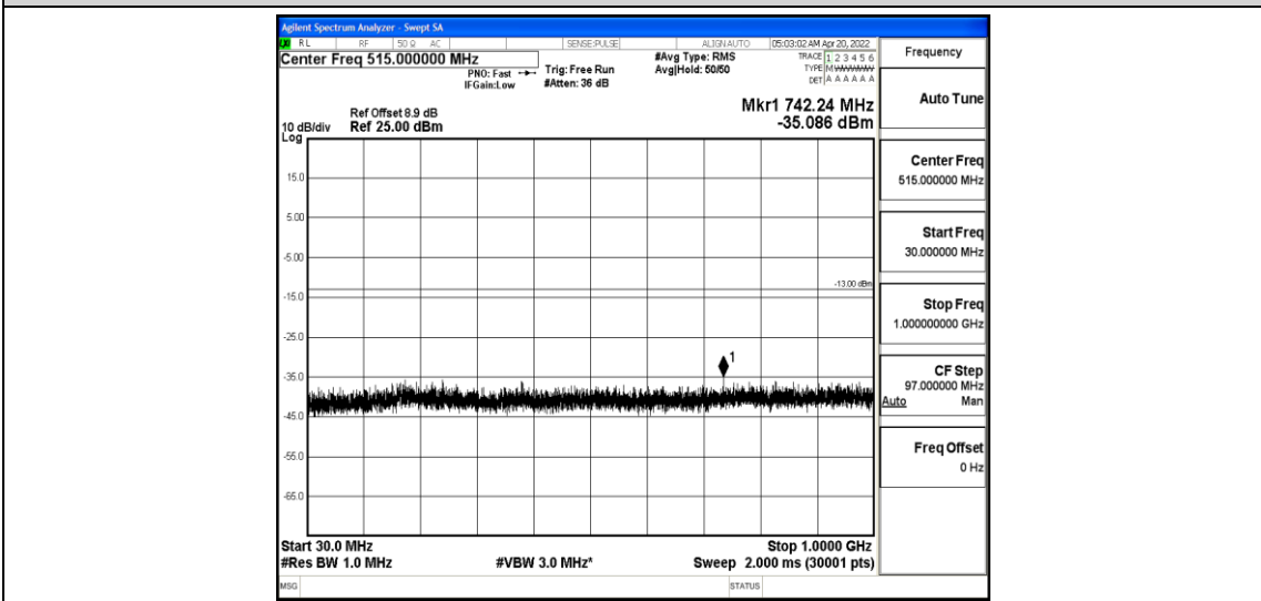
Band25-3MHz-QPSK-26365-1-0-Low-30-1000--35.09-PASS
