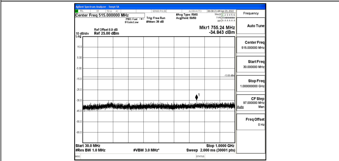
Band25-10MHz-QPSK-26365-1-0-Low-30-1000--34.84-PASS
