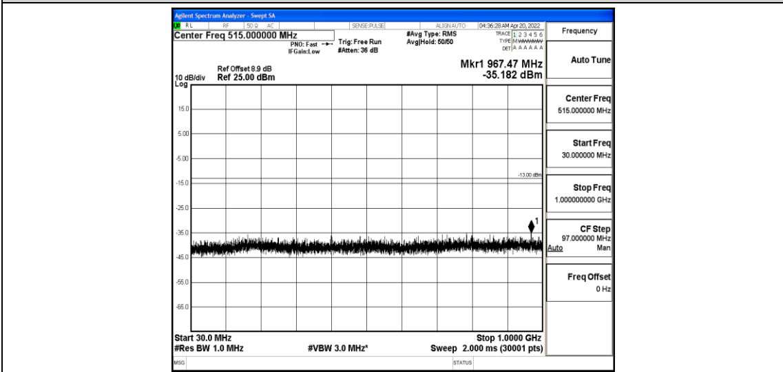
Band25-1.4MHz-QPSK-26365-1-0-Low-30-1000--35.18-PASS
