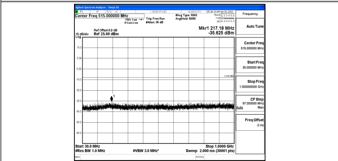
Band25-5MHz-QPSK-26365-1-0-Low-30-1000--35.63-PASS
