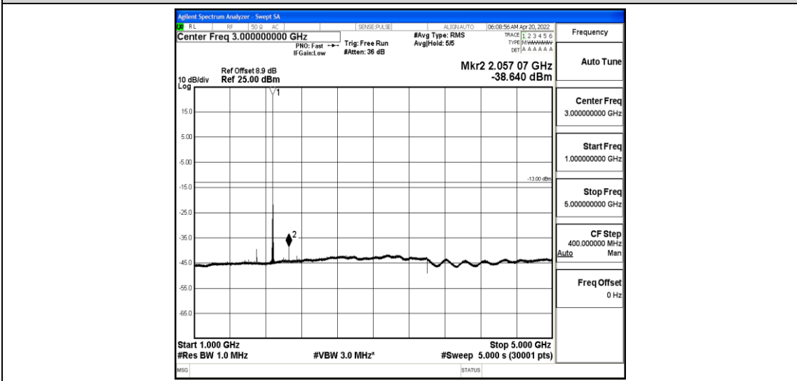
Band25-10MHz-QPSK-26365-1-0-Low-1000-5000--38.64-PASS
