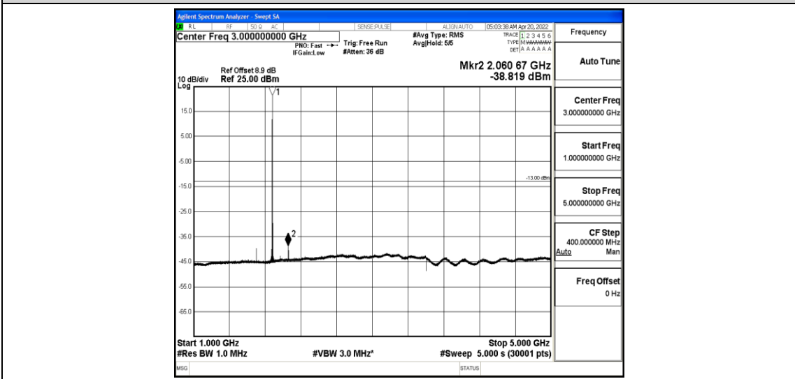
Band25-3MHz-QPSK-26365-1-0-Low-1000-5000--38.82-PASS
