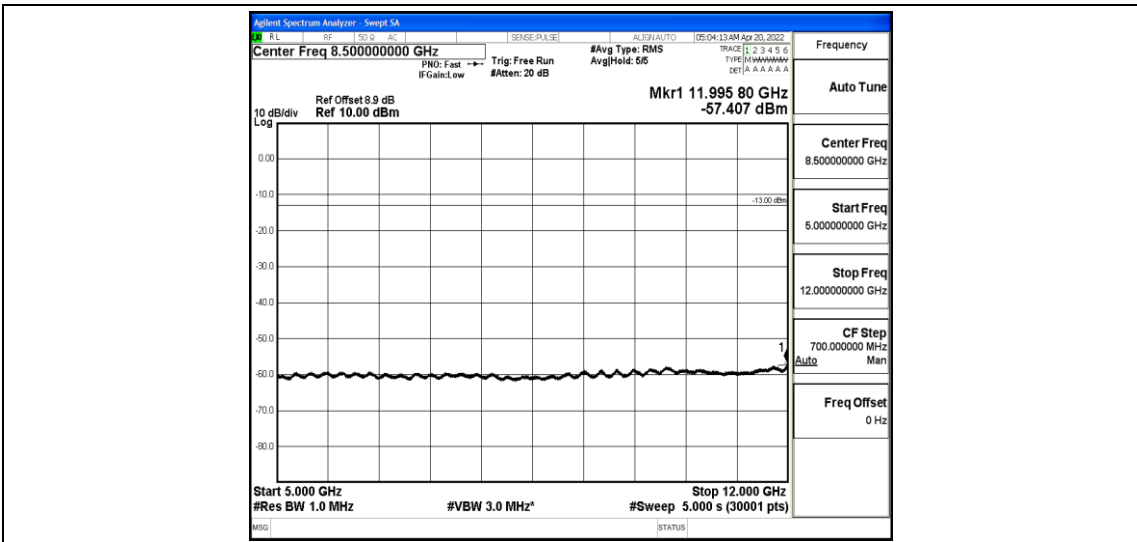
Band25-3MHz-QPSK-26365-1-0-Low-5000-12000--57.41-PASS
