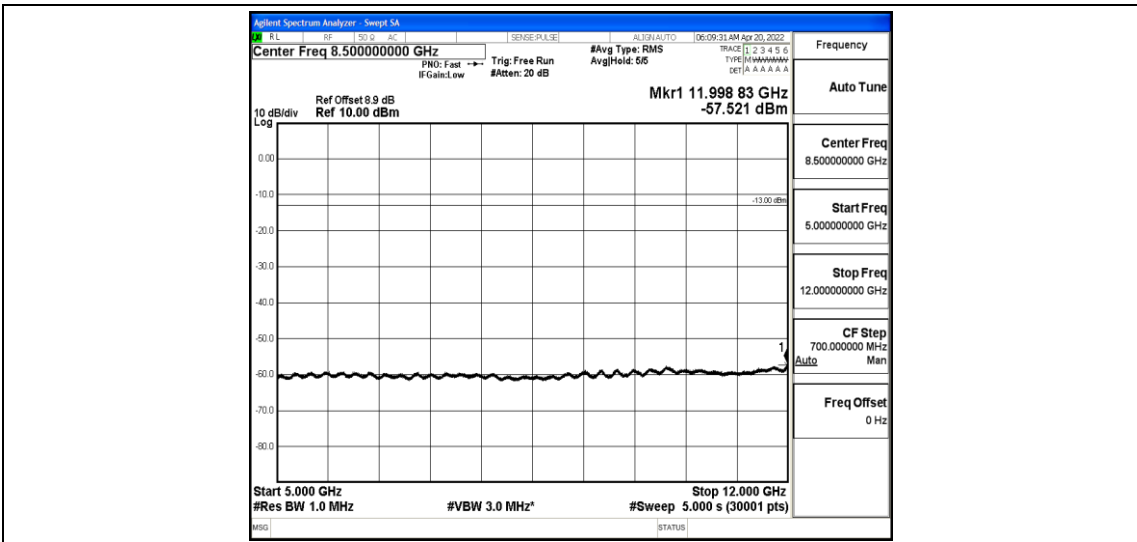
Band25-10MHz-QPSK-26365-1-0-Low-5000-12000--57.52-PASS
