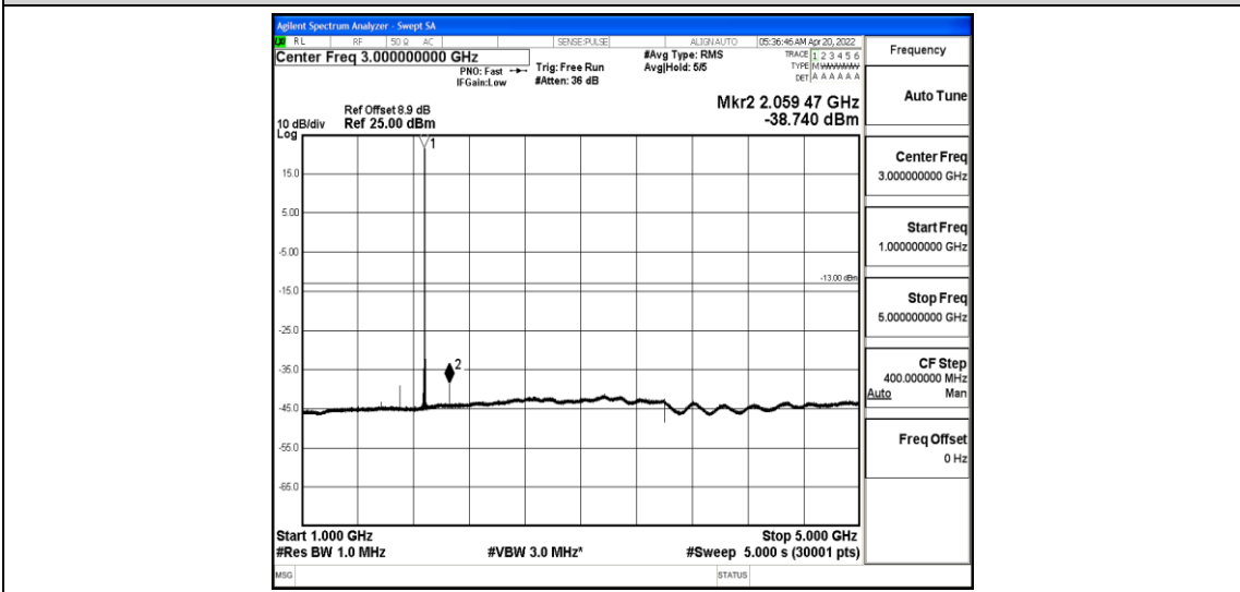
Band25-5MHz-QPSK-26365-1-0-Low-1000-5000--38.74-PASS
