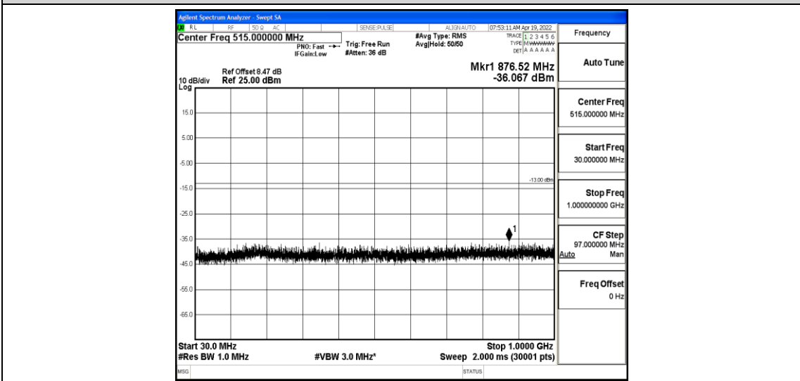
Band4-10MHz-QPSK-20175-1-0-Low-30-1000--36.07-PASS
