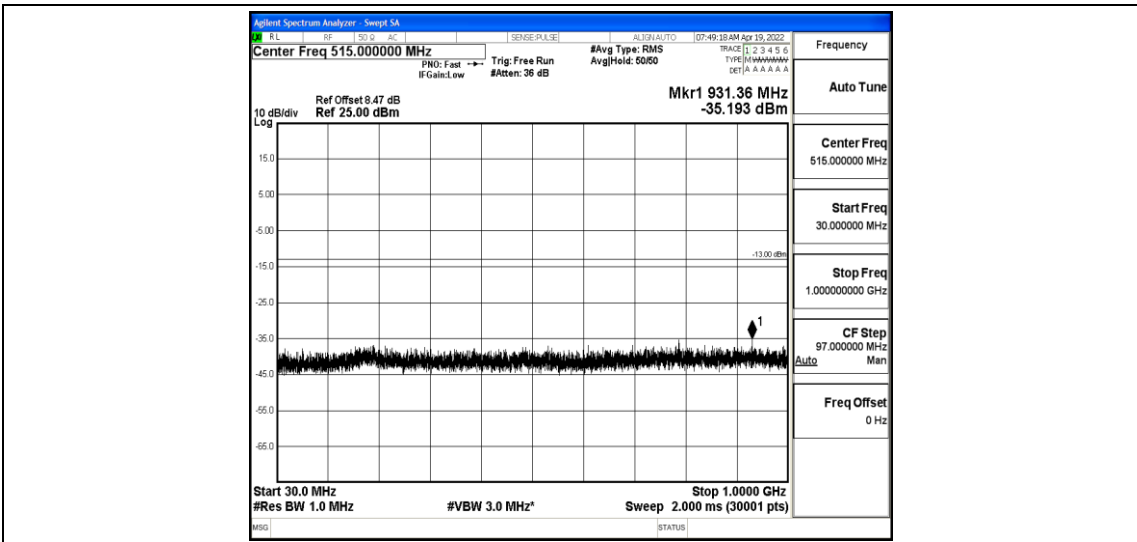
Band4-10MHz-QPSK-20000-1-0-Low-30-1000--35.19-PASS
