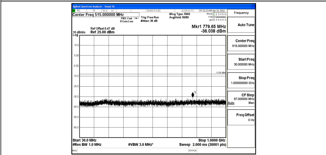
Band4-5MHz-QPSK-20175-1-0-Low-30-1000--36.04-PASS
