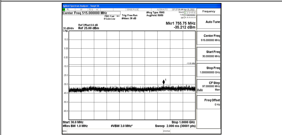
Band2-3MHz-QPSK-18615-1-0-Low-30-1000--35.21-PASS
