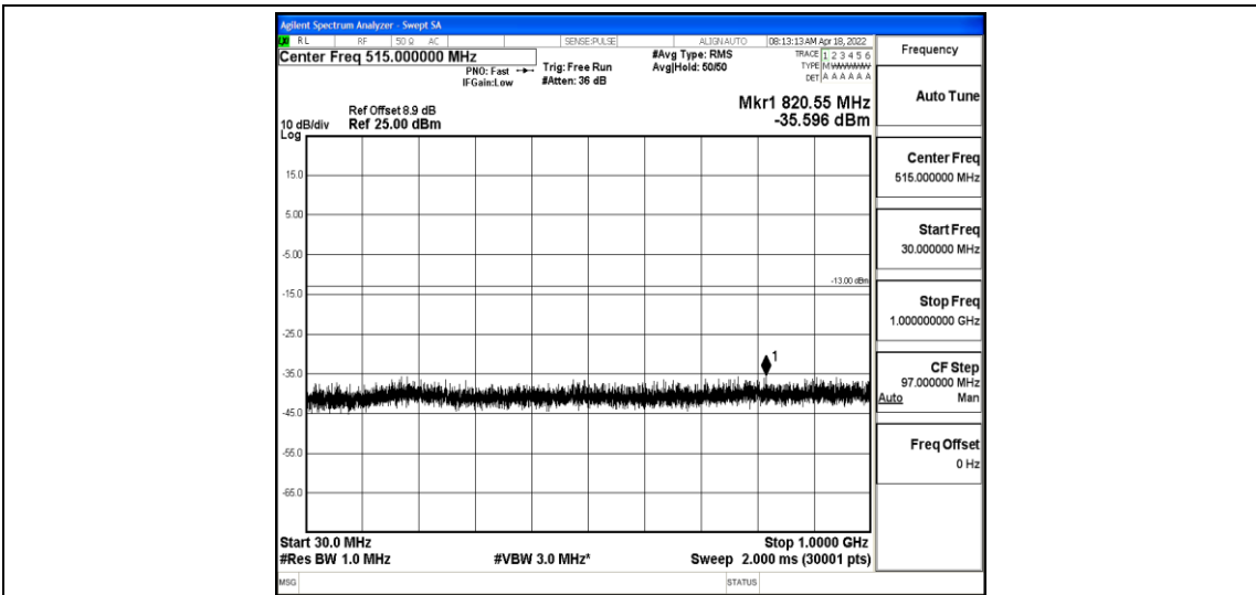
Band2-5MHz-QPSK-18900-1-0-Low-30-1000--35.6-PASS
