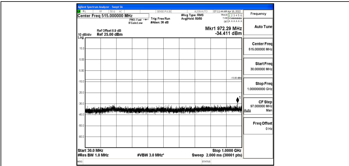
Band2-1.4MHz-QPSK-18900-1-0-Low-30-1000--34.41-PASS
