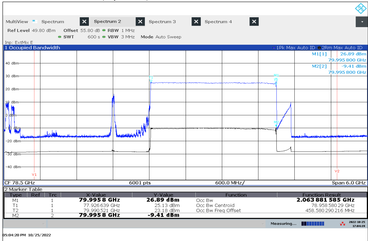
Plot 1: OBW, PSD, T nom / V min-max (City Mode 3)
