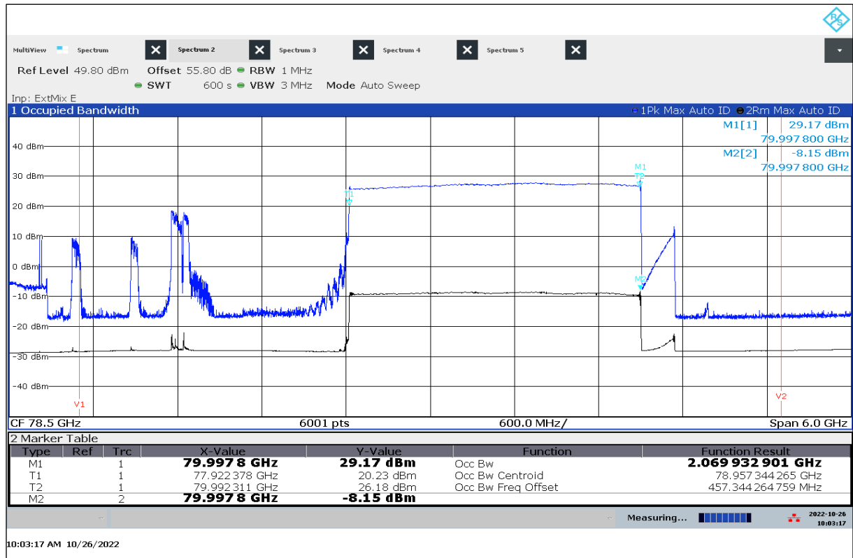
Plot 32: OBW, -20 °C / V nom
