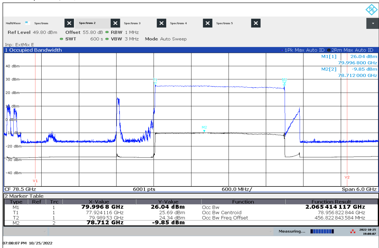
Plot 37: OBW, 30 °C / V nom
