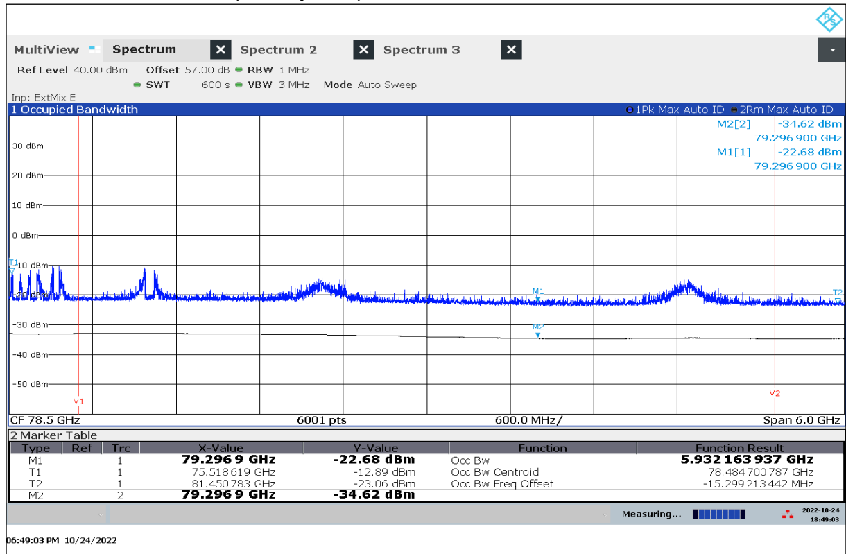
Plot 5: OBW, PSD, T nom / V min-max (StandBy State)
