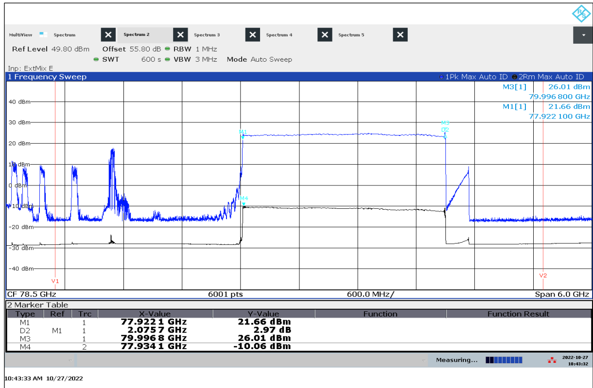
Plot 38: OBW, 40 °C / V nom
