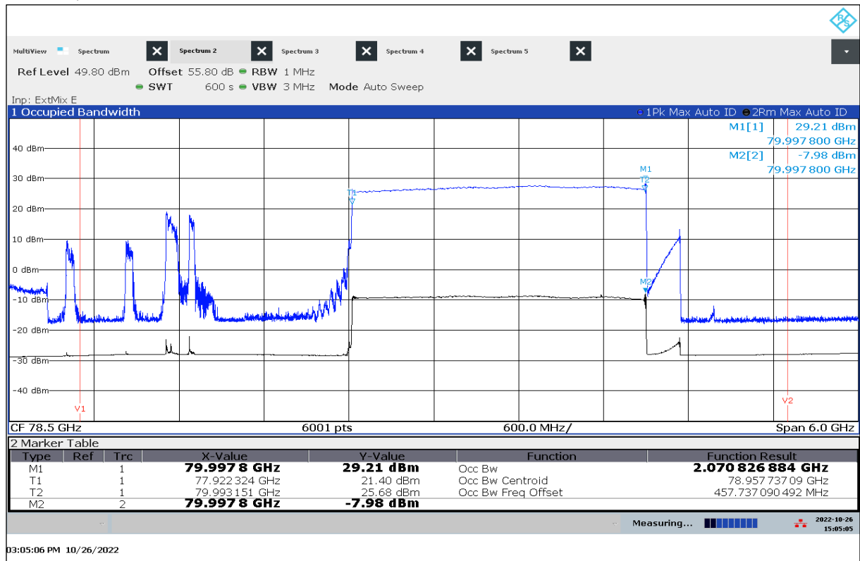
Plot 33: OBW, -10 °C / V nom
