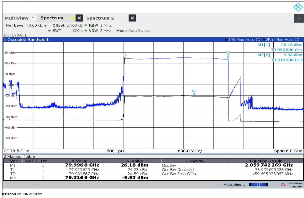
Plot 39: OBW, 50 °C / V nom
