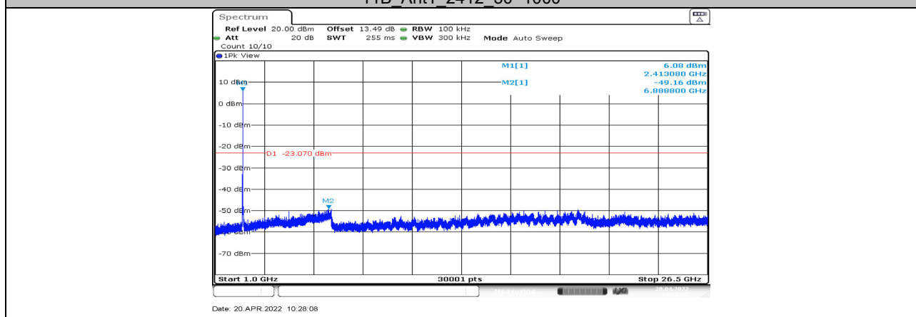
11B_Ant1_2412_1000~26500
