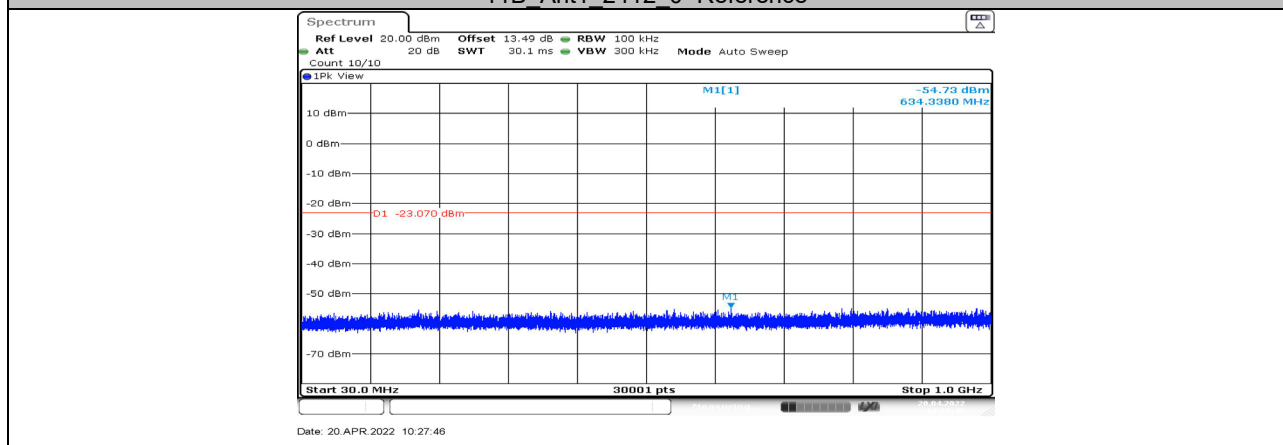
11B_Ant1_2412_30~1000
