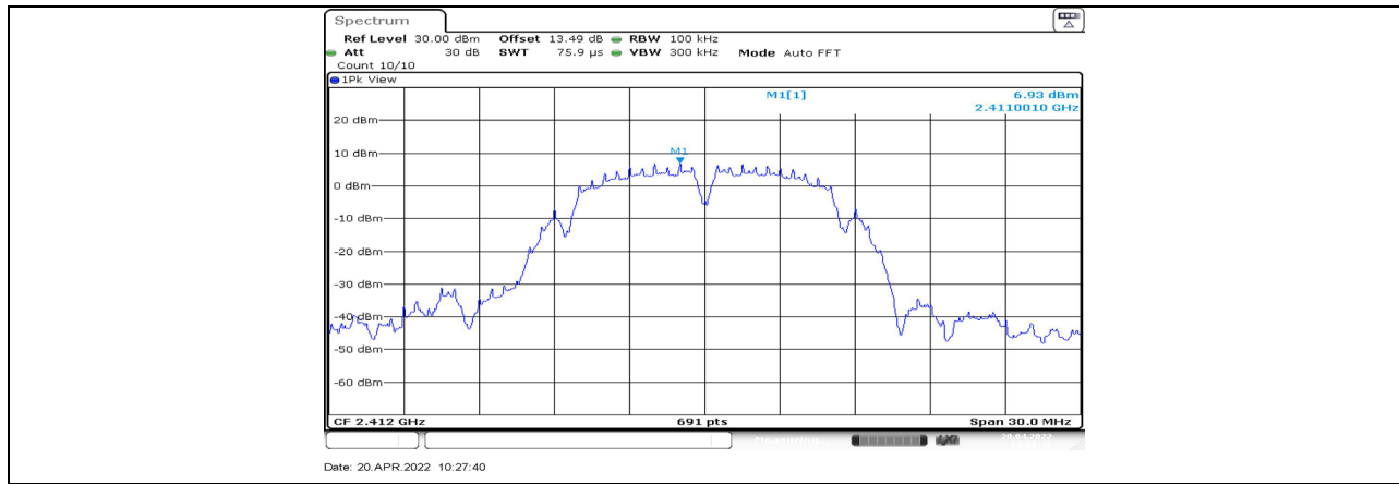
11B_Ant1_2412_0~Reference
