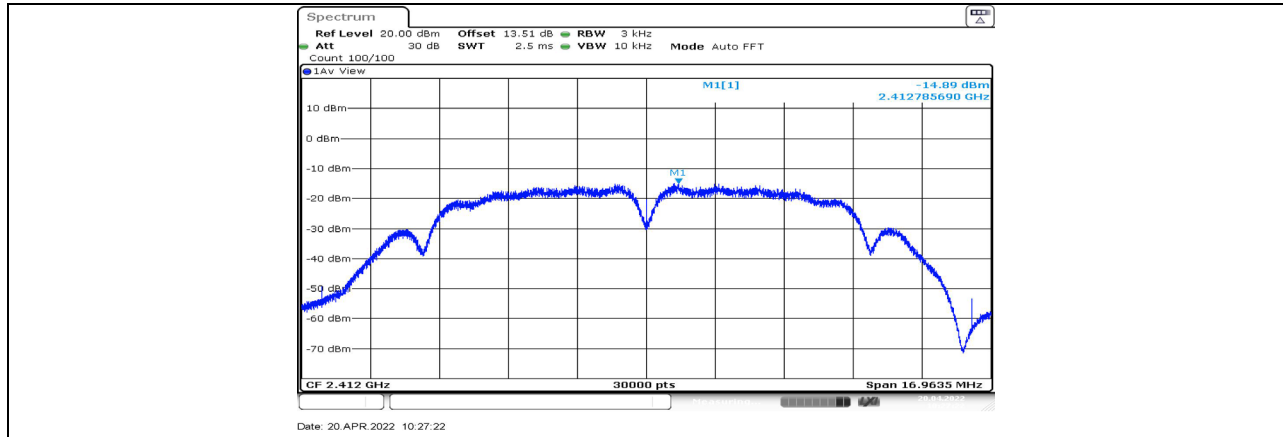
11B_Ant1_2412
