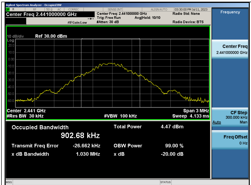
Test_Graph_ANT1_2441_1Mbps_OBW
