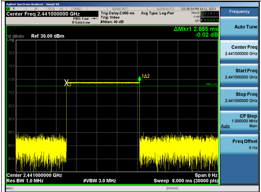
Test_Graph_HOP_ANT1_NA_1Mbps_2441_Time per Burst
