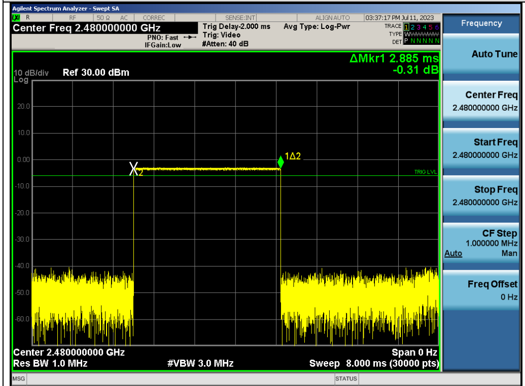
Test_Graph_HOP_ANT1_NA_1Mbps_2480_Time per Burst
