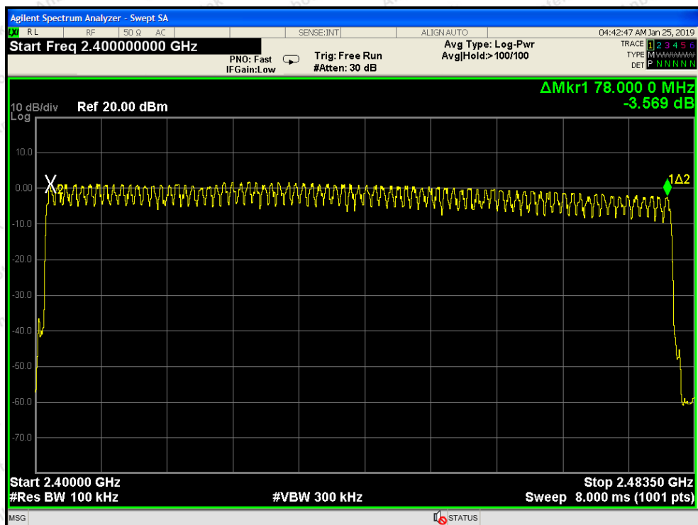
EDR Mode(8DPSK)
