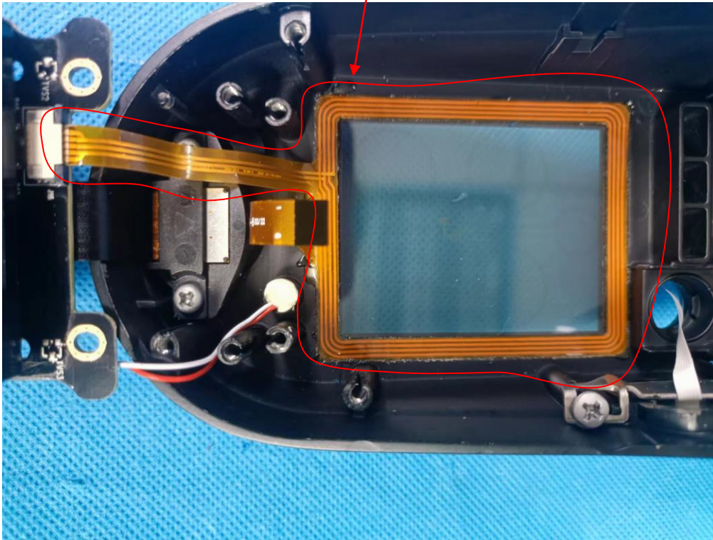
RFID antenna
