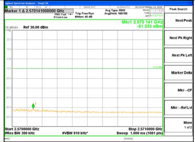
2570-2571MHz
