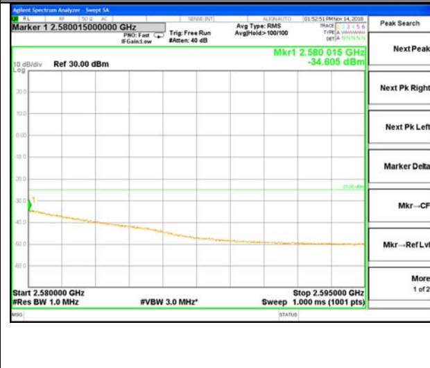
2580-2595MHz
