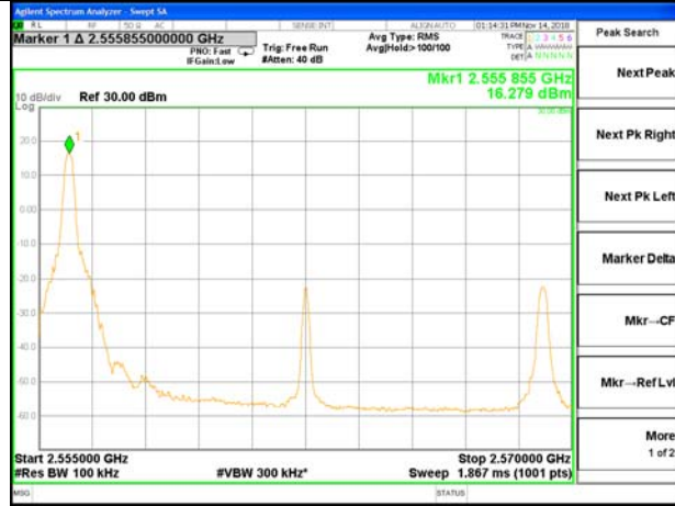
2555-2570MHz
