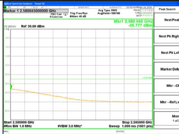
2580-2595MHz
