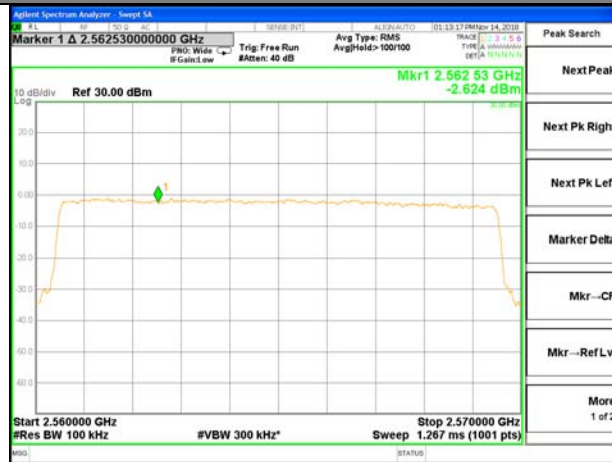
2560-2570MHz
