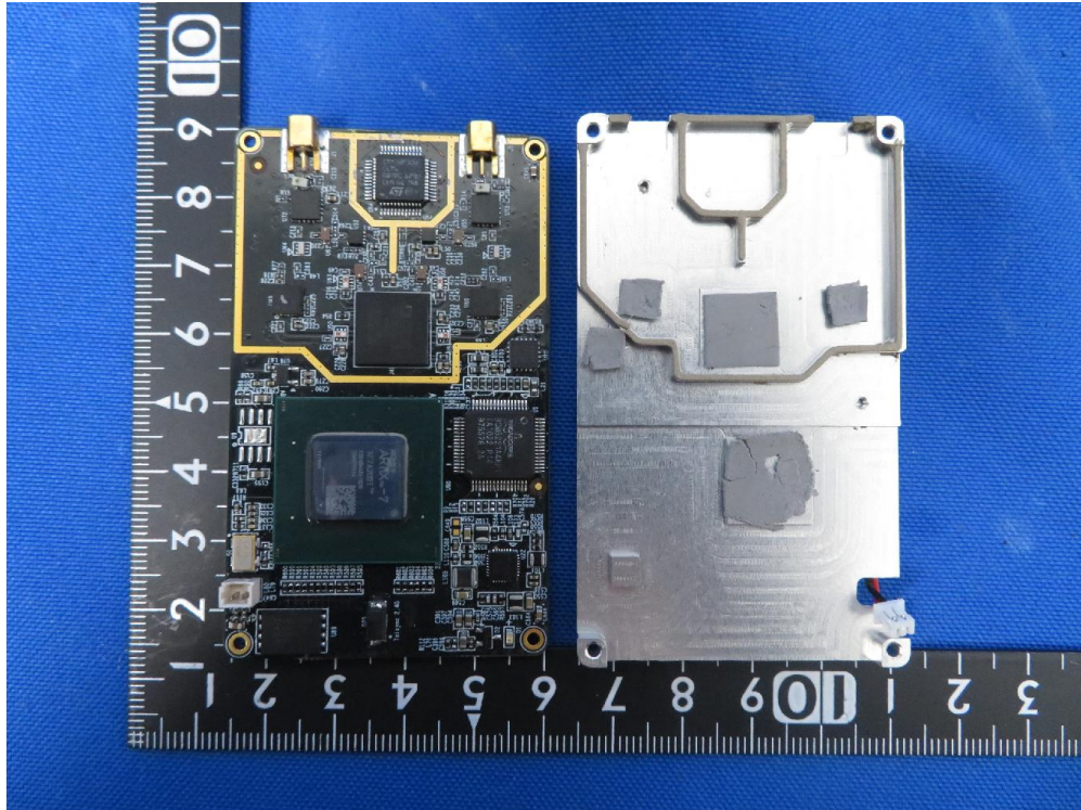
(1) EUT Photo (Model: IAUS11901a)
