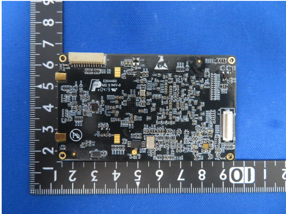
(5) EUT Photo (Model: IAUS11901a)
