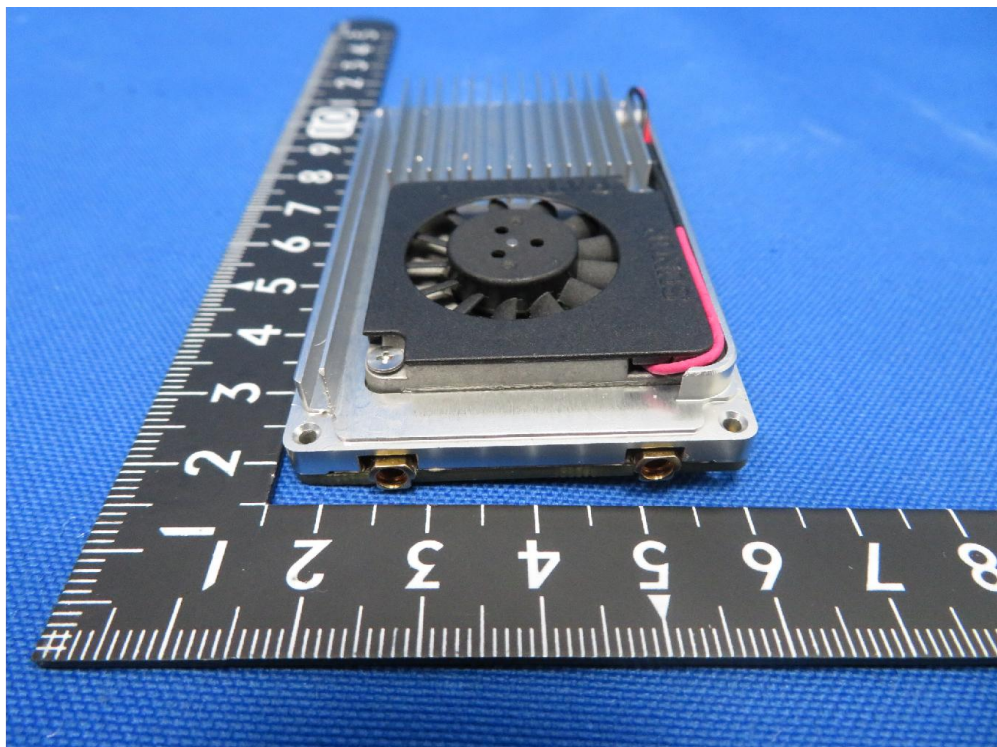
(4) EUT Photo (Model: IAUS11901a)
