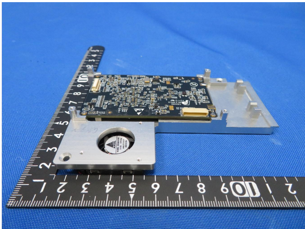
(14) EUT Photo (Model: IAUS11901c)
