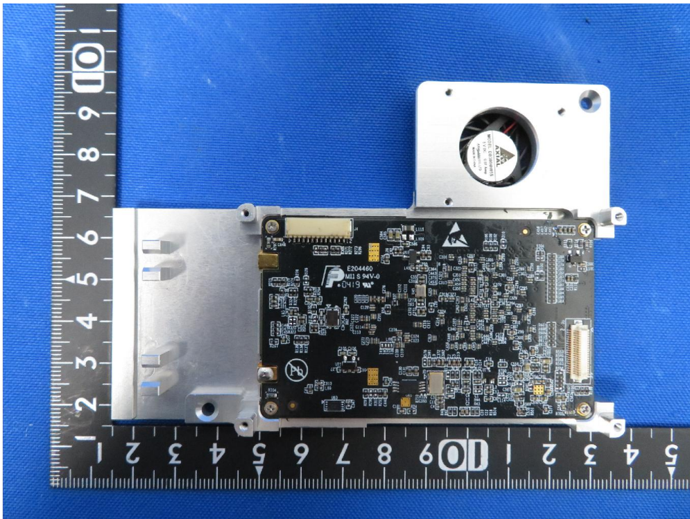
(12) EUT Photo (Model: IAUS11901c)
