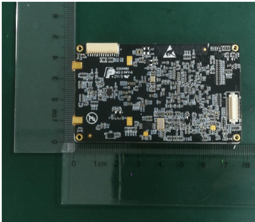
(10) EUT Photo (Model: IAUS11901b)
