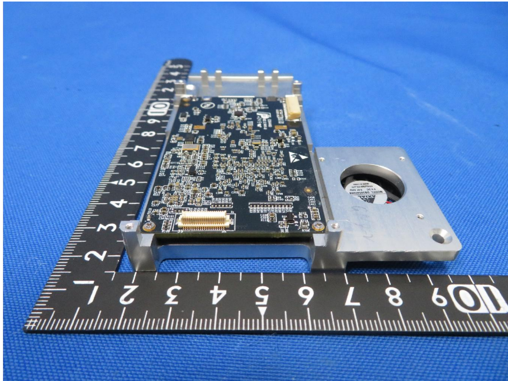
(15) EUT Photo (Model: IAUS11901c)
