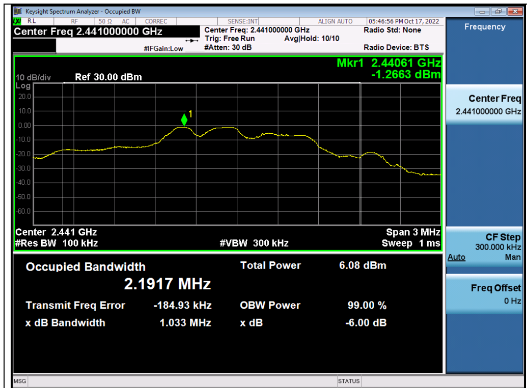
Test_Graph_GFSK_ANT1_2441_DTSBW
