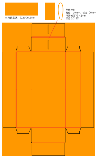
内盒黑底157g双胶+吸胶
