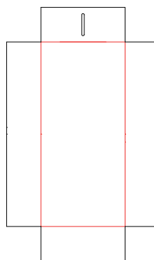
内盒1000g单面白, V槽90度
