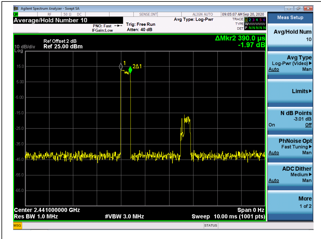
(DH1, 8-DPSK)
