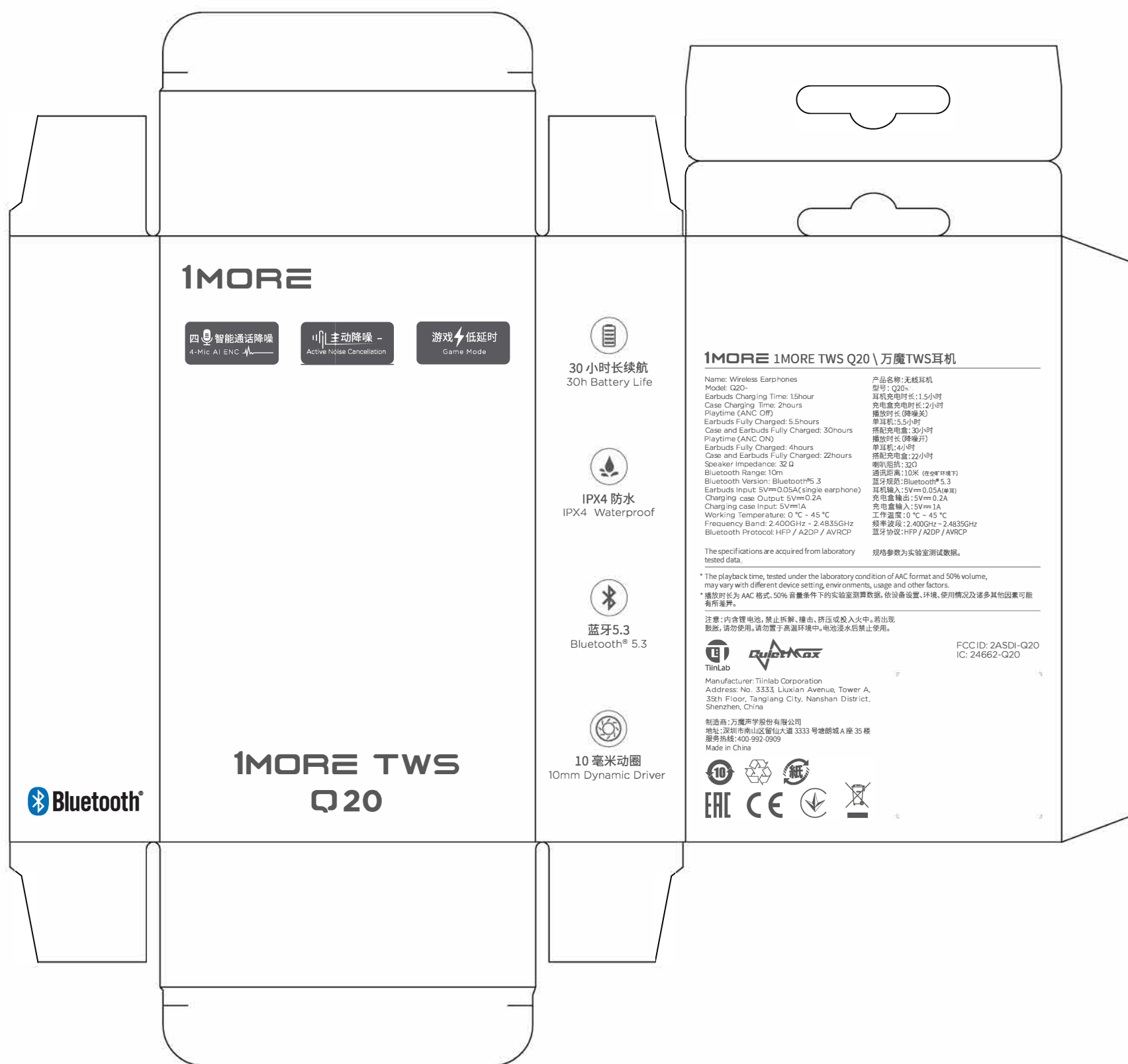
烫银示意图
