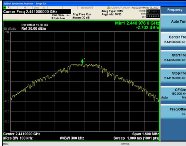
DH5-Ant1-2441-30~1000--2.70
