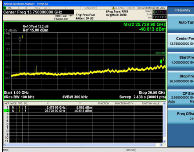
3DH5-Ant1-2480-0-Reference-5.51
