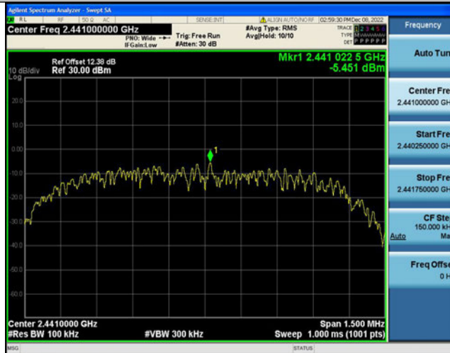
2DH5-Ant1-2441-30~1000--5.45
