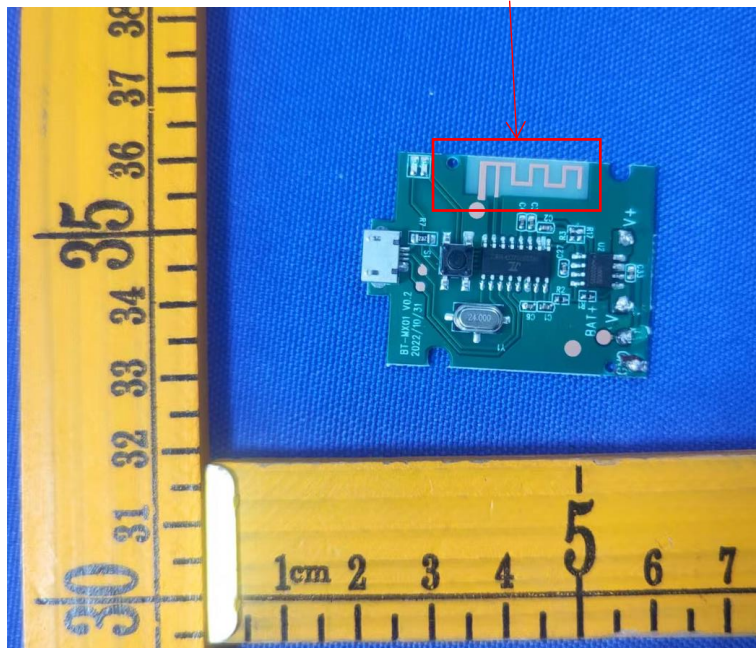
Antenna
