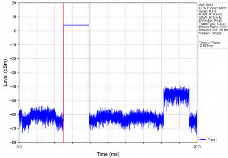
GFSK_DH5_HOPP_Ant1_NTV
