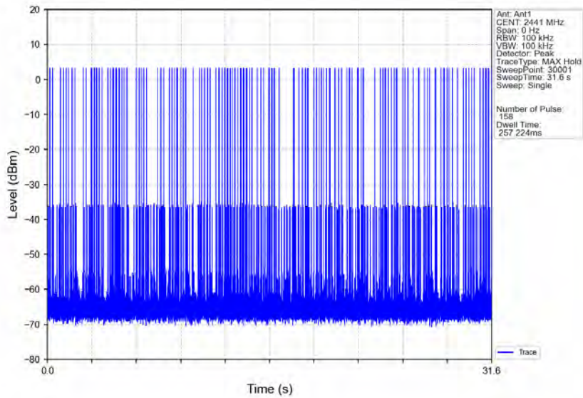
GFSK_DH3_HOPP_Ant1_NTV
