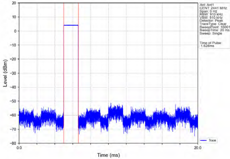
GFSK_DH3_HOPP_Ant1_NTV
