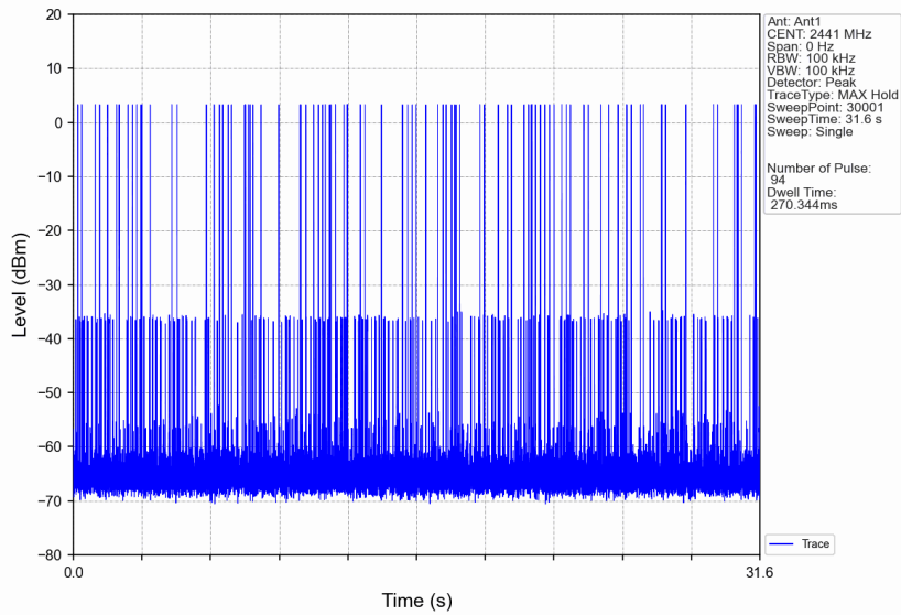
GFSK_DH5_HOPP_Ant1_NTV
