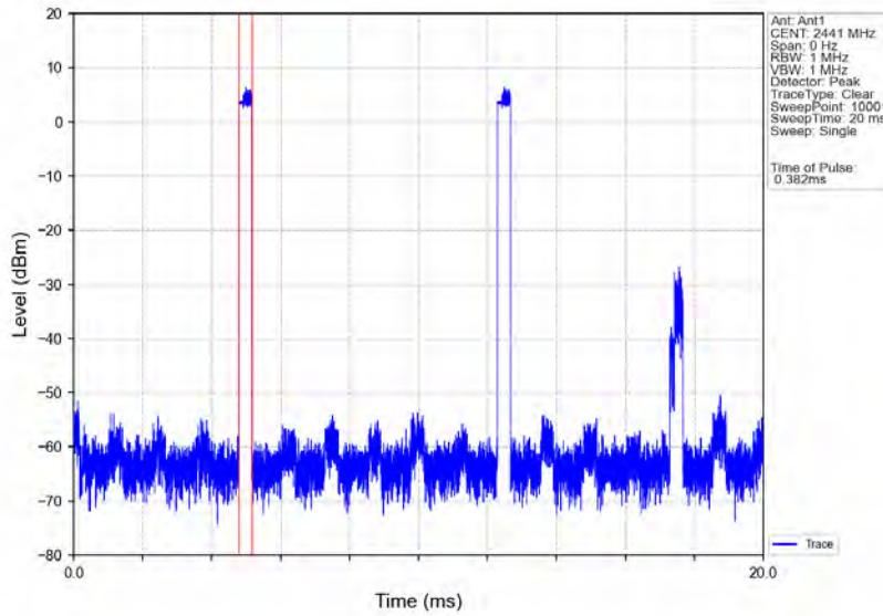
8DPSK_3DH1_HOPP_Ant1_NTNV
