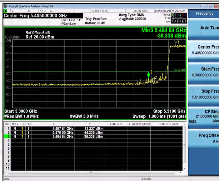
11AX20SISO_Ant1_Low_5500
