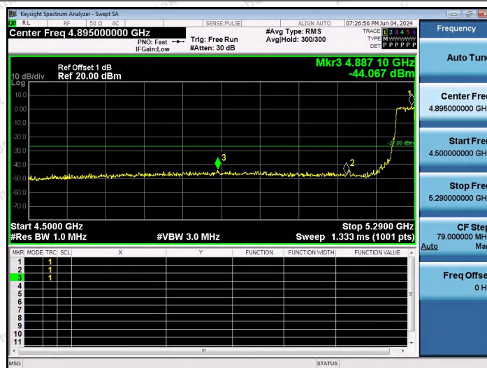
11N40SISO-Ant1-5270-PASS
