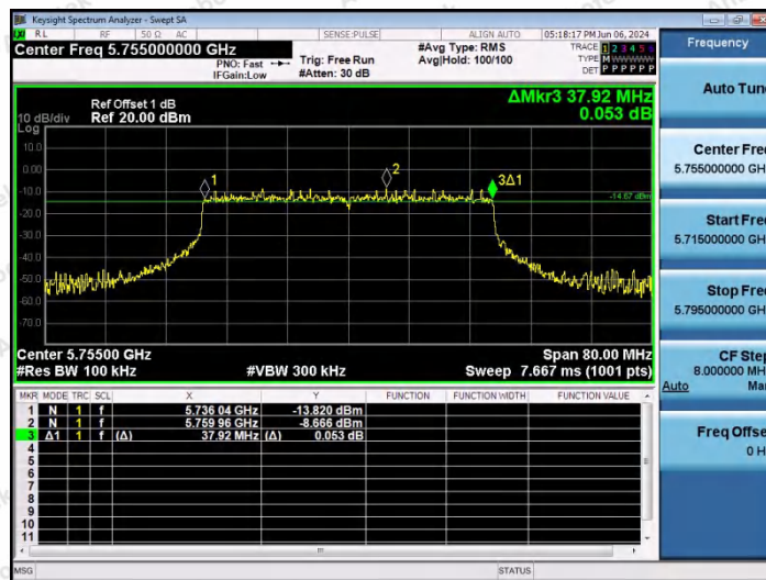
11AX40ISO-Ant1-5755-PASS
