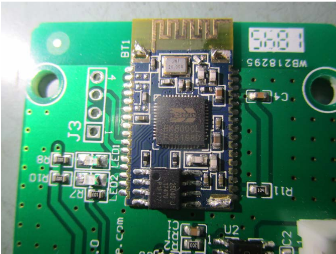
BT module
