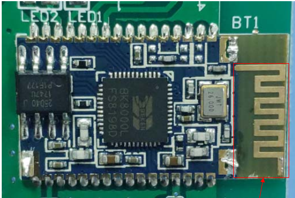
2.4G Antenna
