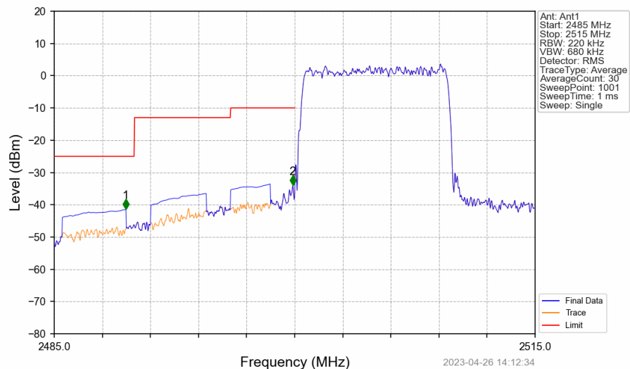
Band7 10MHz 16QAM LCH 2505MHz RB 50 0 NTNV
