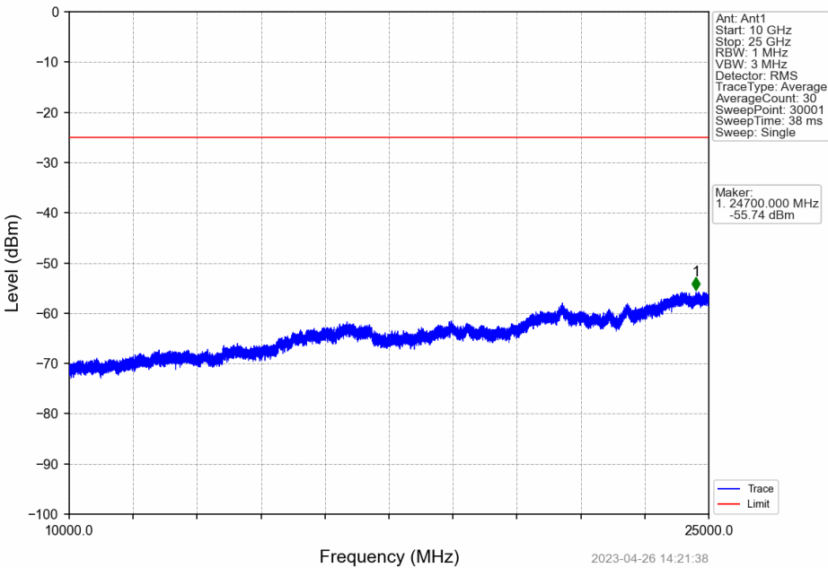
Band7 20MHz 16QAM MCH 2535MHz RB 1 0 NTNV
