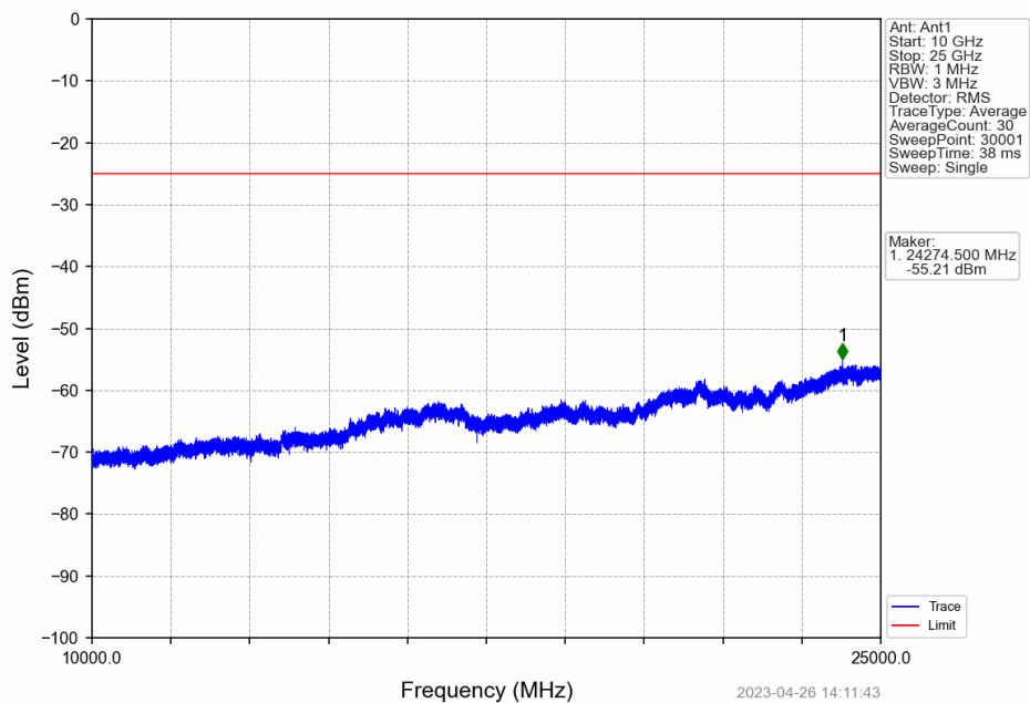
Band7 10MHz QPSK LCH 2505MHz RB 1 0 NTV
