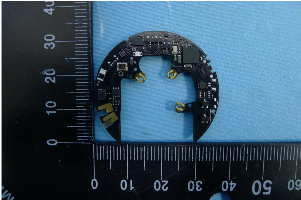
(10) EUT Photo
