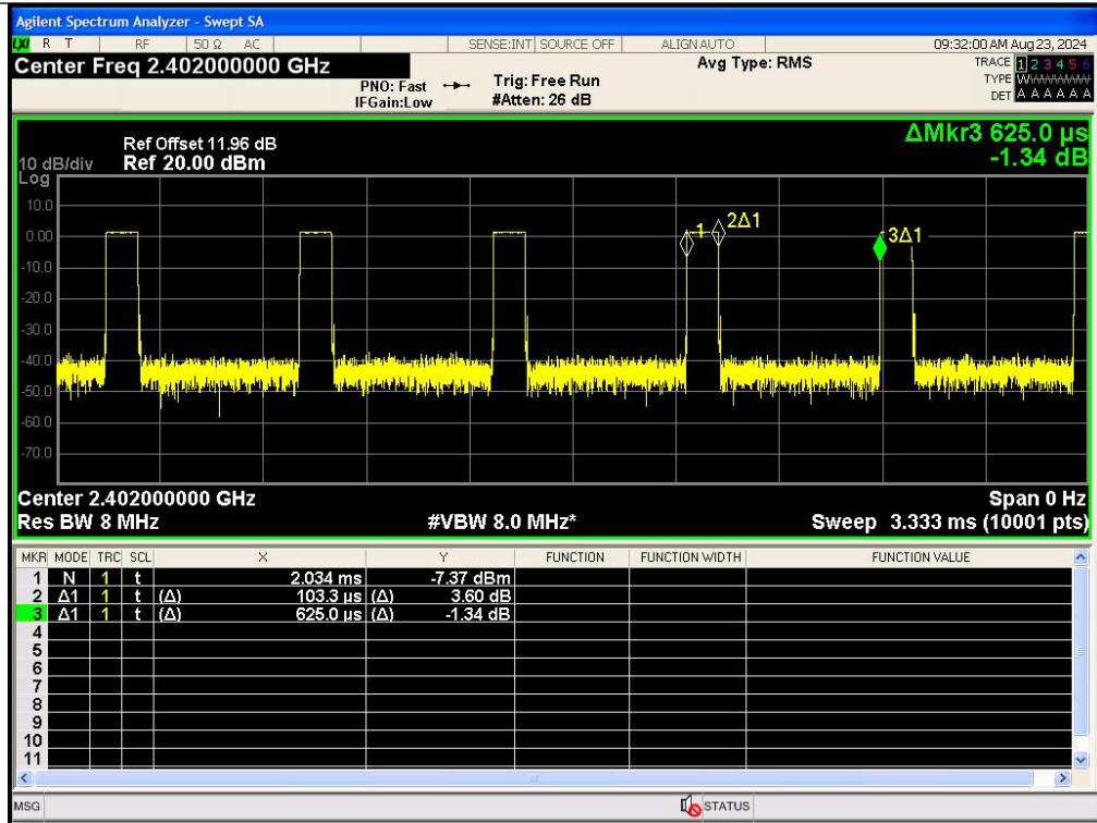
BLE 1M_Channel 0
