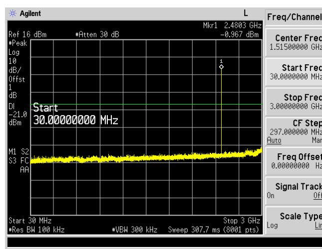
30MHz-3GHz
