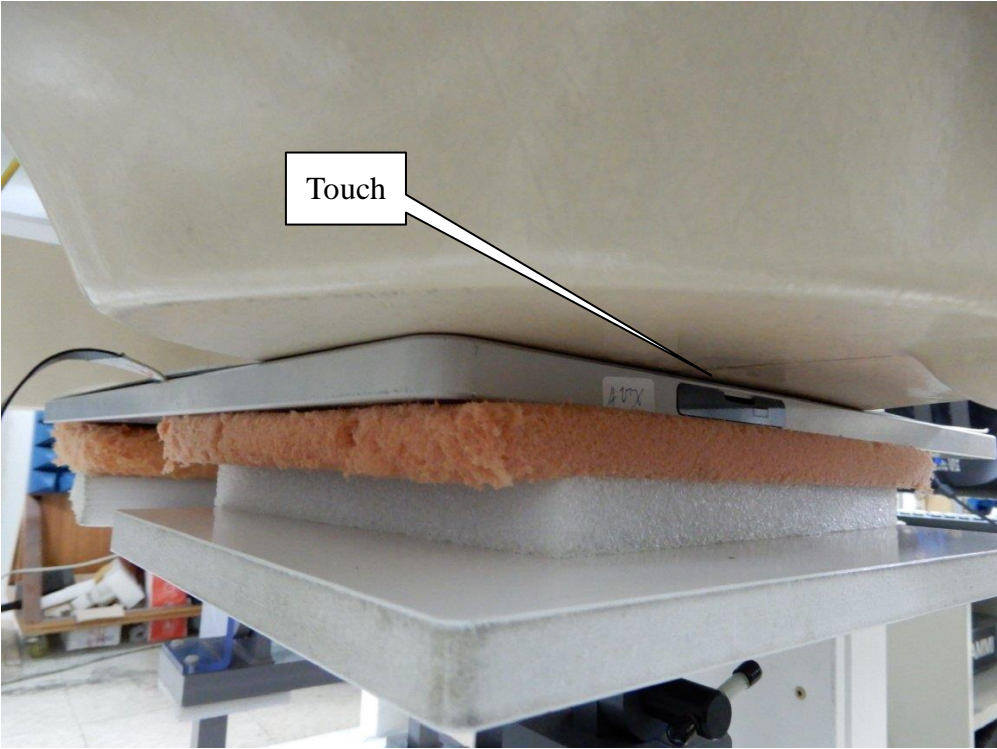
EUT Front – Body SAR (Aux Antenna)
