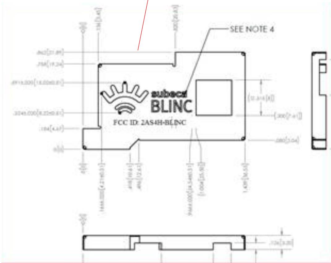
EUT Label Position
