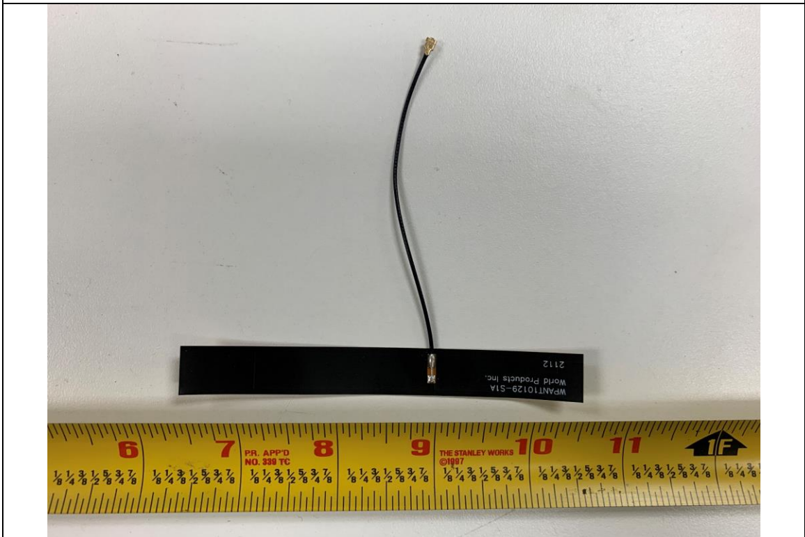
LoRA antenna
