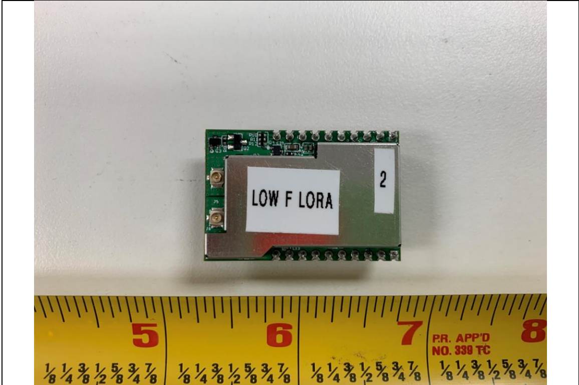
EUT External-Front
