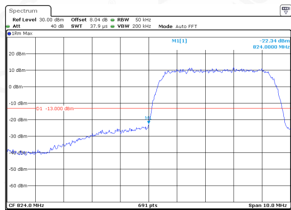
WCDMA 850-LCH
