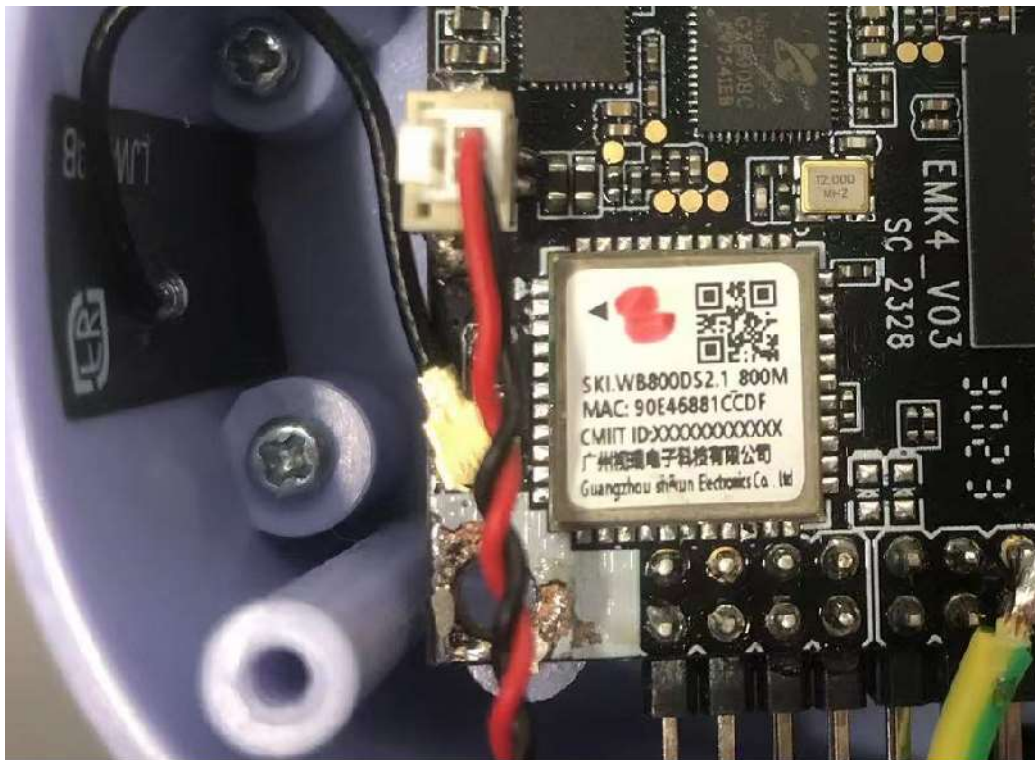
WiFi module
