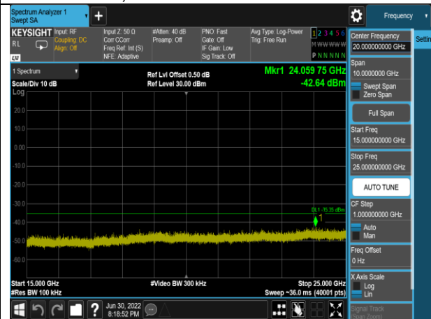
802.11n(HT40),2452MHz,Ant0,Plot 6,15000MHz~25000MHz
