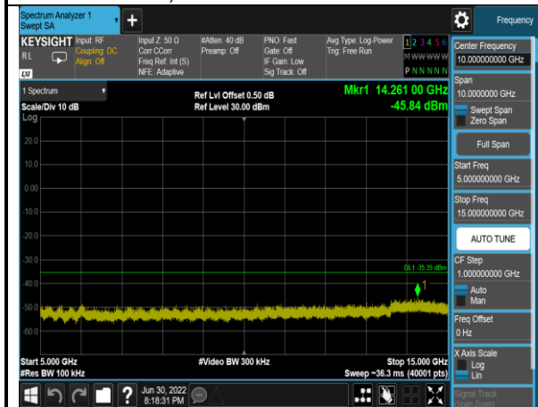
802.11n(HT40),2452MHz,Ant0,Plot 5,5000MHz~15000MHz
