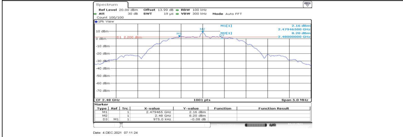
ZIGB_Ant1_2480
