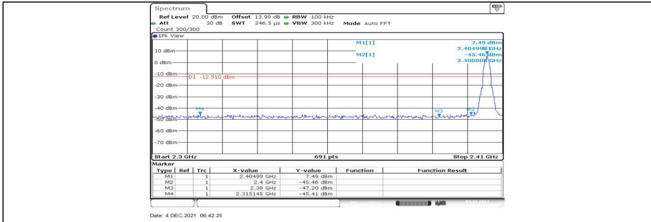
ZIGB_Ant1_Low_2405
