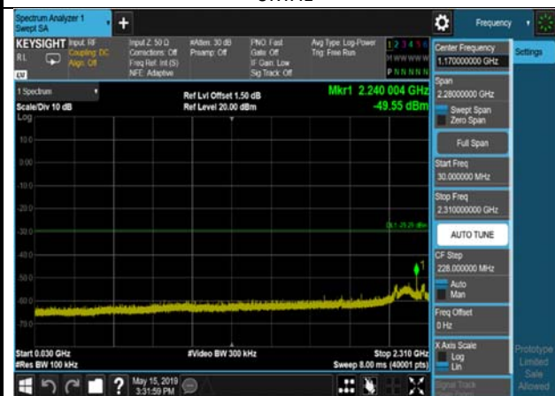
802.11g,2437MHz,Ant0,Plot 3,30MHz~2310MHz
