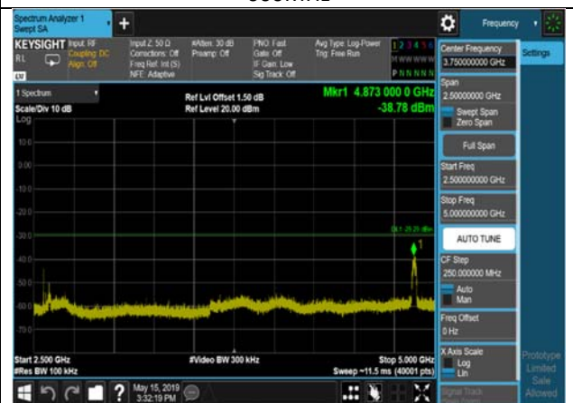
802.11g,2437MHz,Ant0,Plot 4,2500MHz~5000MHz
