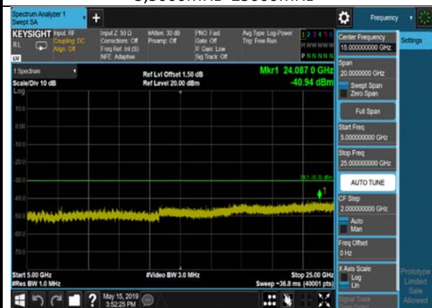
802.11n(HT20),2412MHz,Ant0,Plot 5,5000MHz~25000MHz
